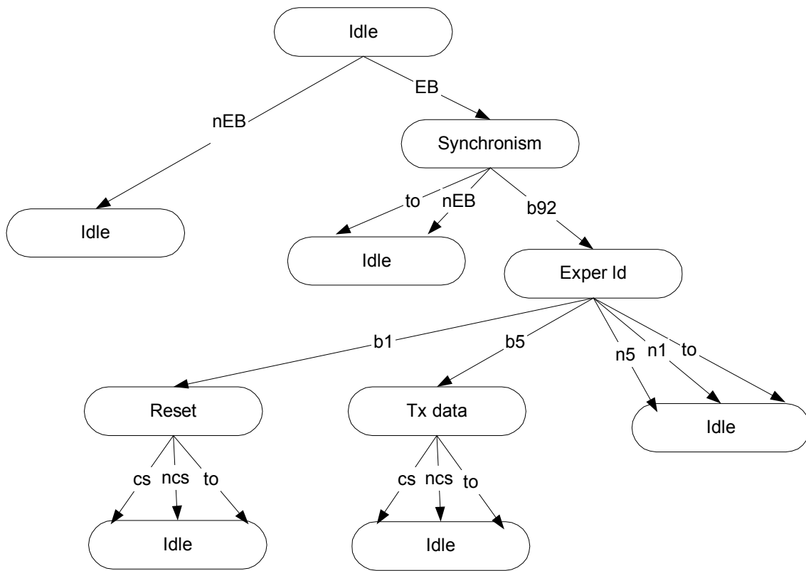
FIGURA B.7 - Árvore de alcançabilidade da N+ para OBDDH-Exp 2comandos.
