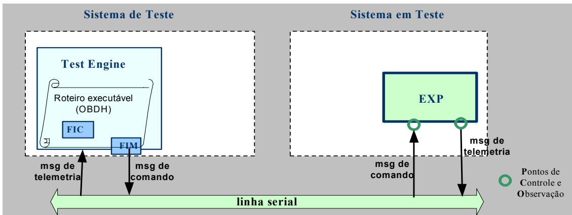
FIGURA 4.7 - Arquitetura Ferry-injection para teste do OBDR-EXP.
