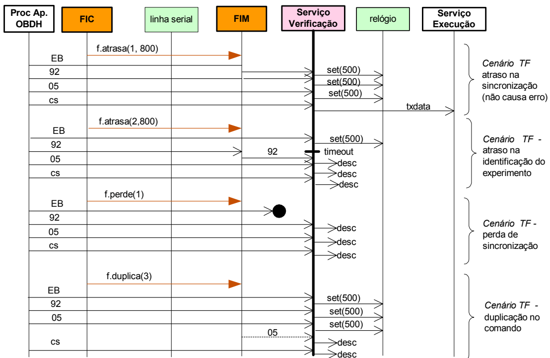
FIGURA 4.12 - Diagrama de Seqüência Exceções de TF OBDH-EXP.
