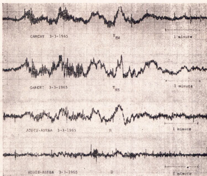
Fig. 2 — La microstructure moyenne (3 mars) est bien marquée à Garchy sur les deux composantes; elle est nette sur H à Addis mais faible sur D. La microstructure fine, nettement marquée à Garchy sur les deux composantes, n'apparaît que sur H à Addis et les oscillations sont moins nombreuses.
