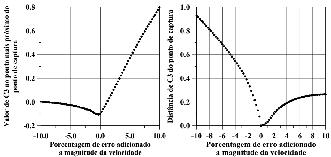
Fig. 9.6 – Resultados para erros de 10% na magnitude da velocidade.
