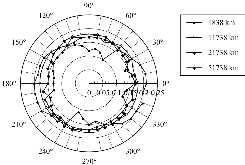
Fig. 6.4 – Valores mínimos de C3 para vários r_p na captura direta.
