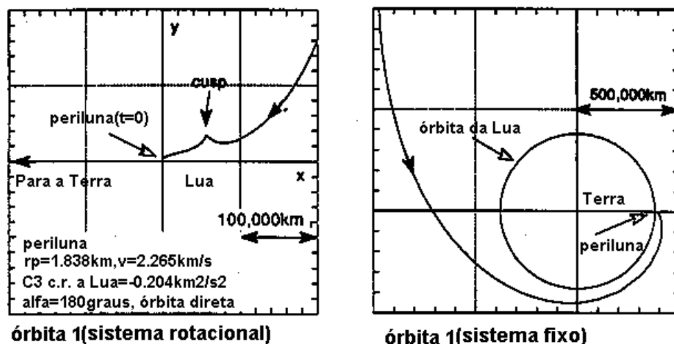
Fig. 3.4 – Figura 3-24 de Yamakawa (1992).
