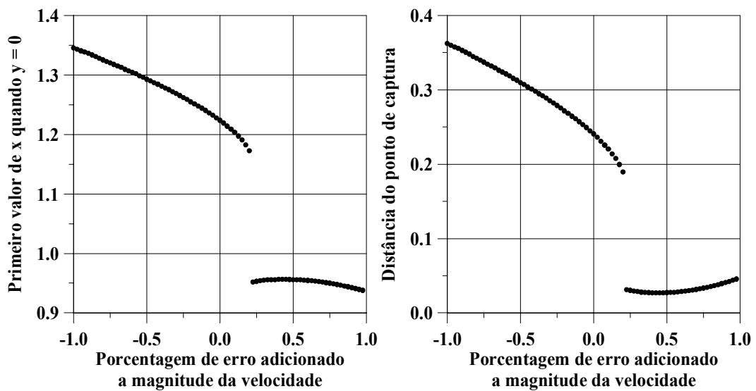
Fig. 9.15 – Resultados para erros de 1% na magnitude da velocidade.
