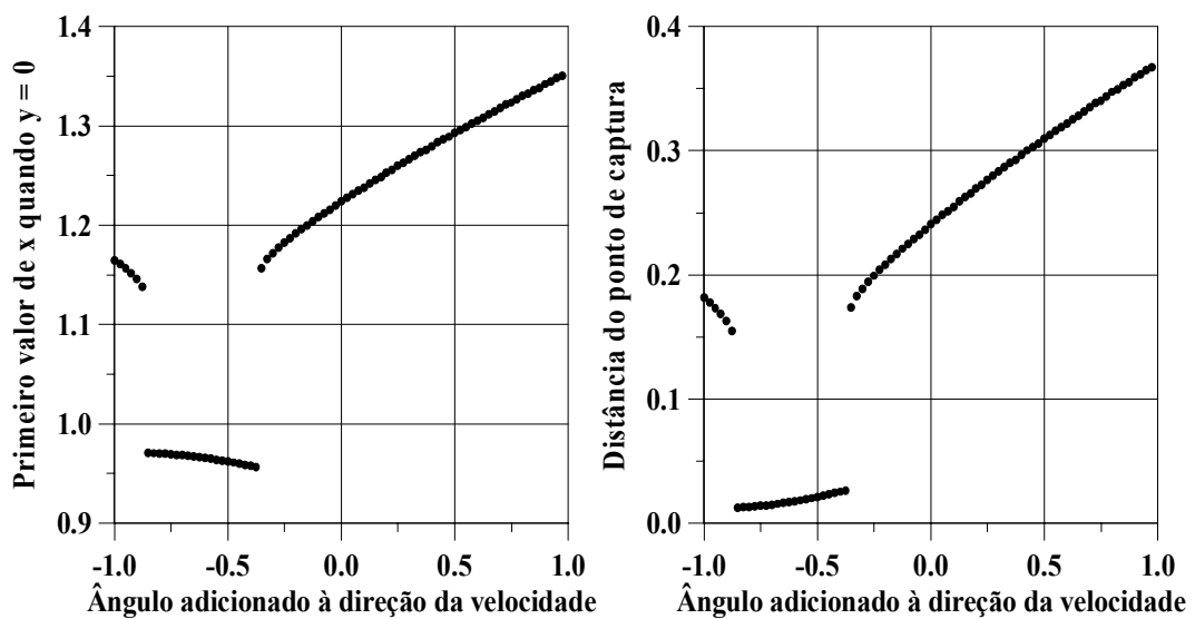
Fig. 9.28 – Resultados para erros de até 1° na direção da velocidade.
