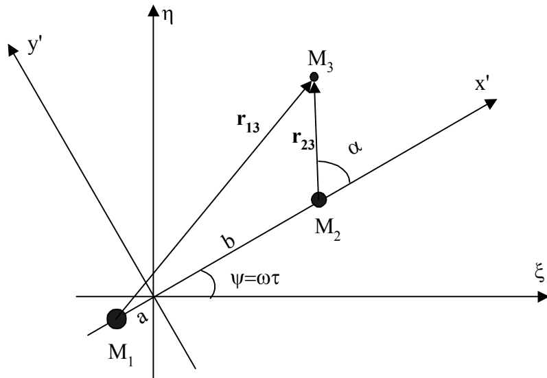
Fig. 2.1 – Sistema de coordenadas (inercial, \xi - \eta , e rotacional, x' - y' ) para o problema restrito circular de três corpos.
