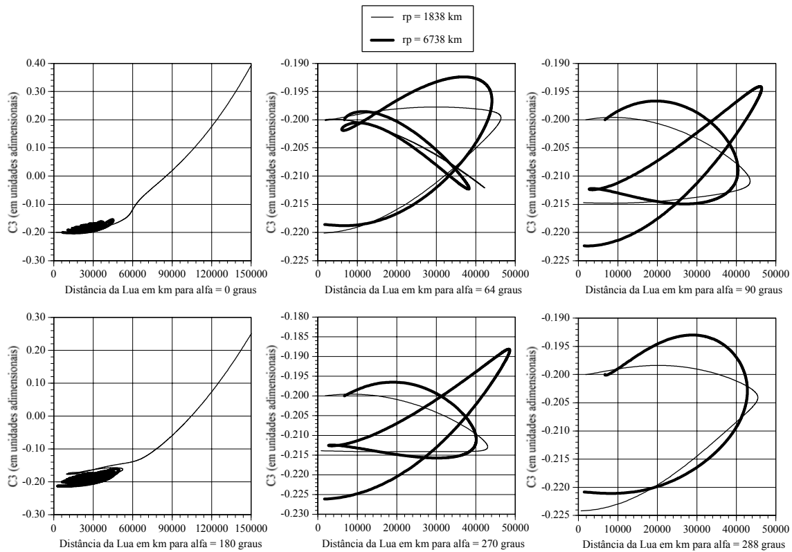
Fig. 4.3 – Comportamento de C_3 em relação à distância da Lua para o valor inicial de C_3 = -0.2 .
