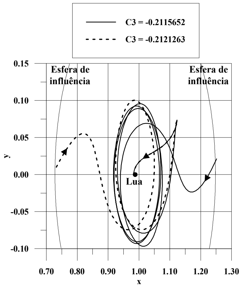
Fig. 3.9 – Trajetórias que produzem a descontinuidade entre \beta = 5^\circ e \beta = 178.8^\circ .
