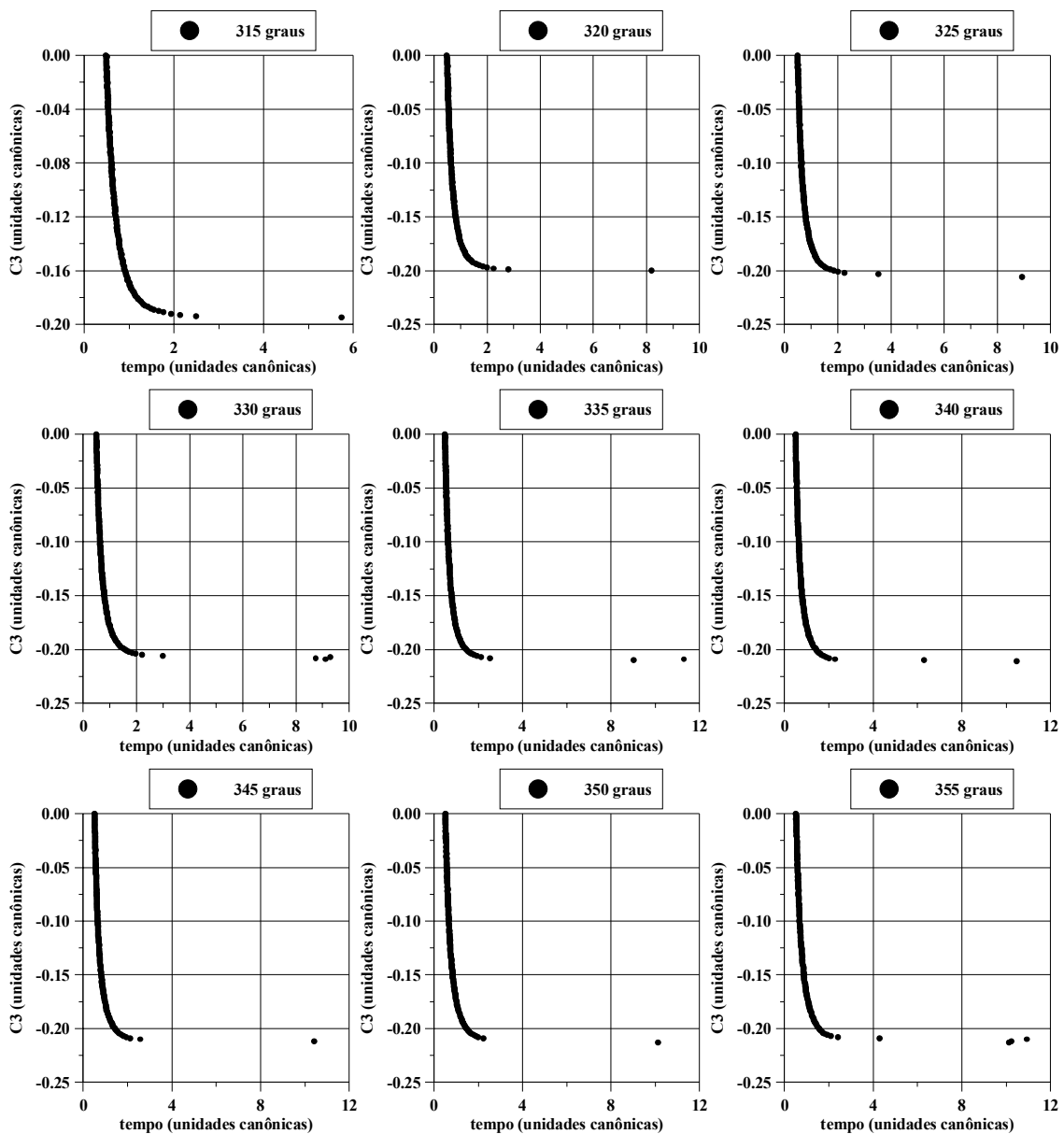
Fig. 7.3 – Tempo de captura vs. C3. (Conclusão).
