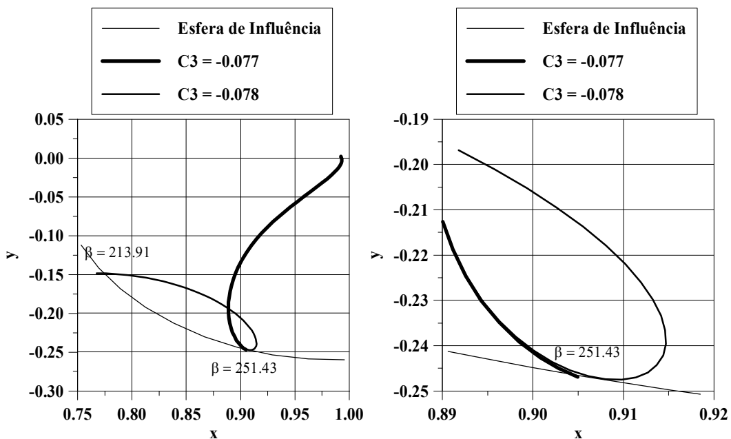
Fig. 7.4 – Trajetórias que provocam a descontinuidade do ângulo \alpha = 25^\circ da Figura 7.3.
