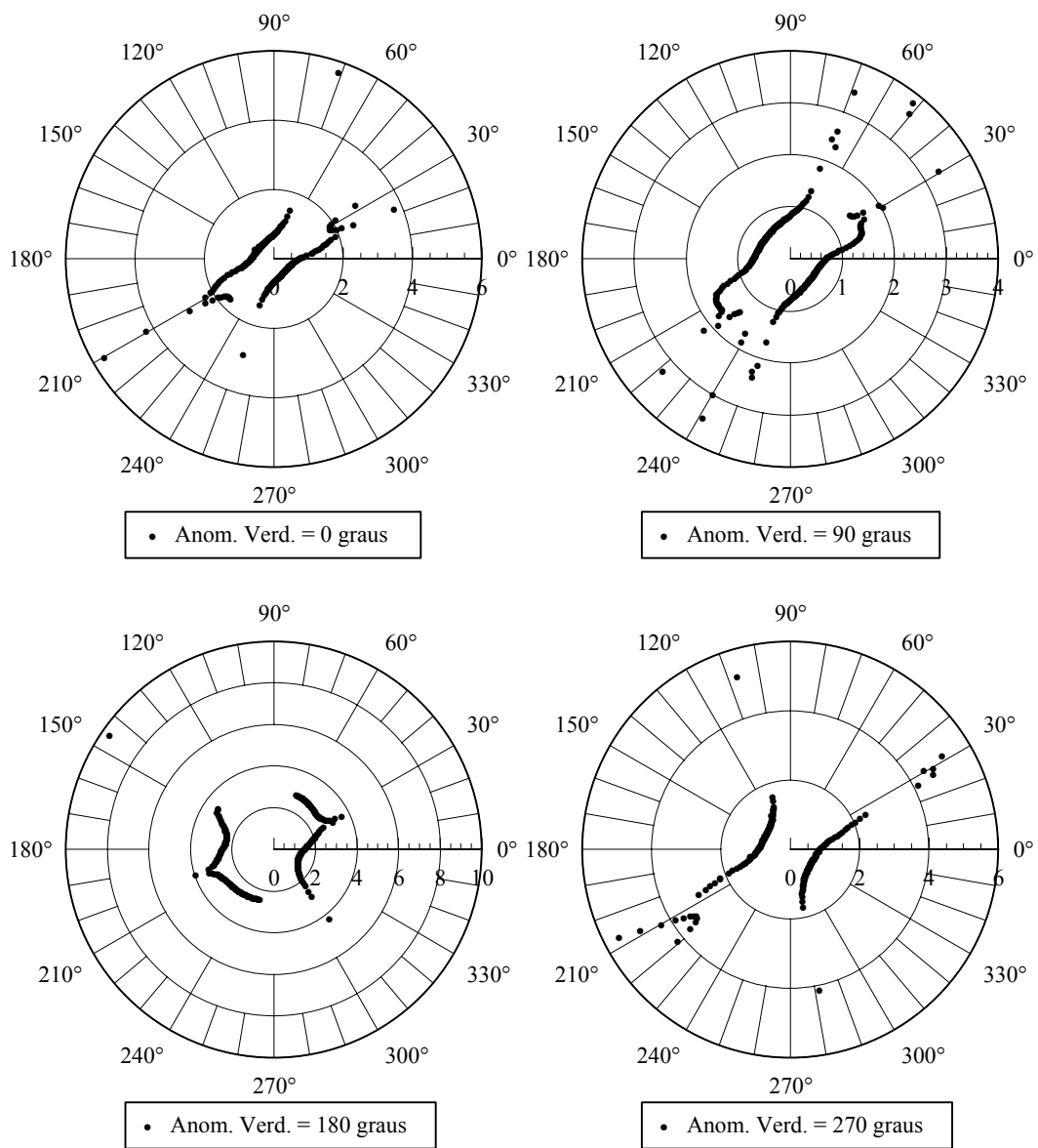
Fig. 8.7 – Tempos de captura para excentricidade de 0.4.
