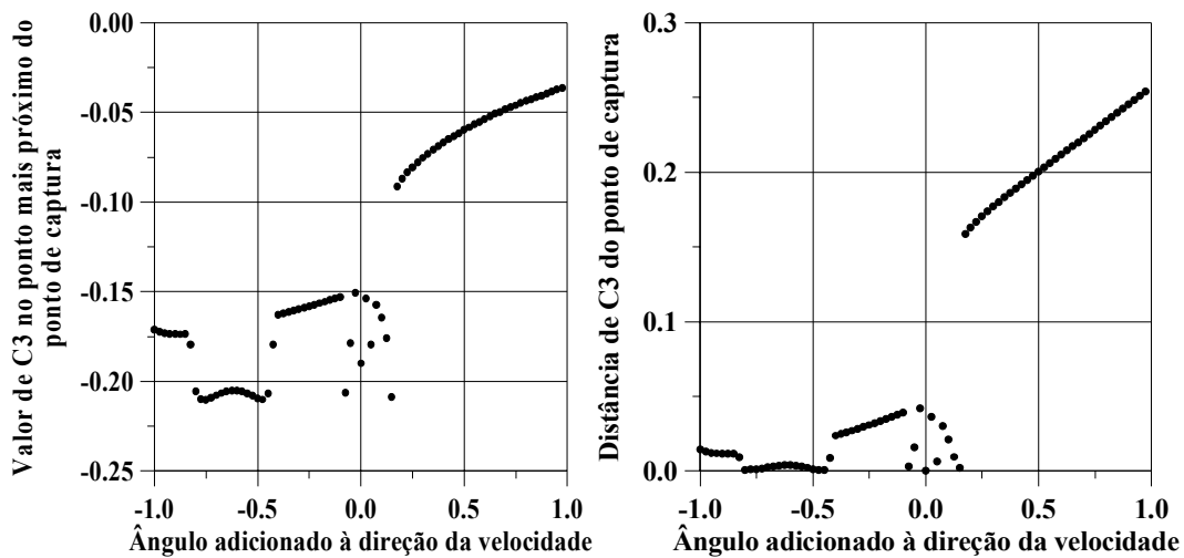
Fig. 9.29 – Resultados para erros de até 1^\circ na direção da velocidade.
