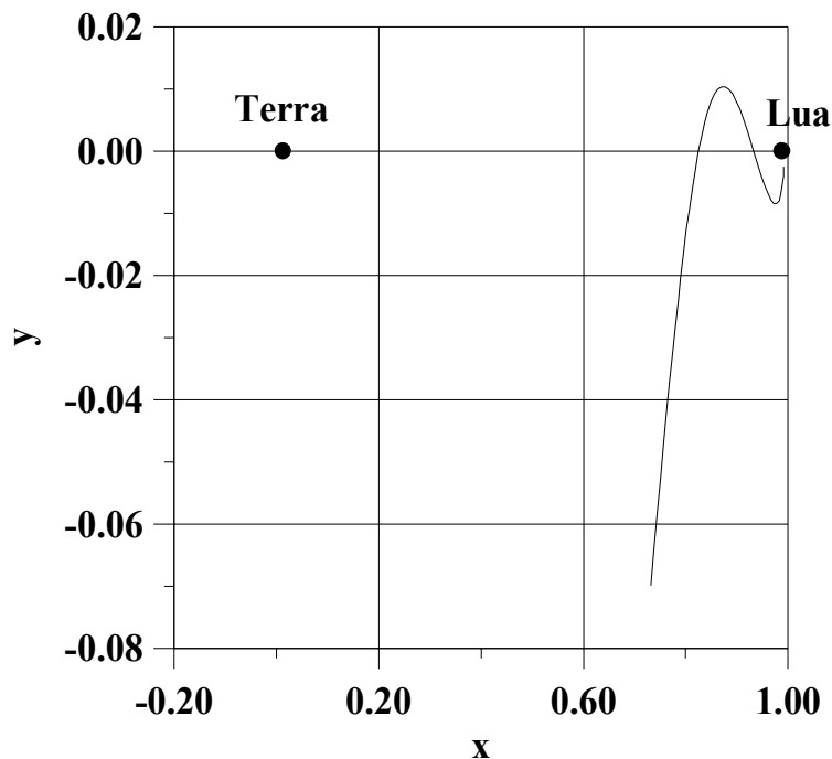
Fig. 8.10 – Trajetória do problema 2.
