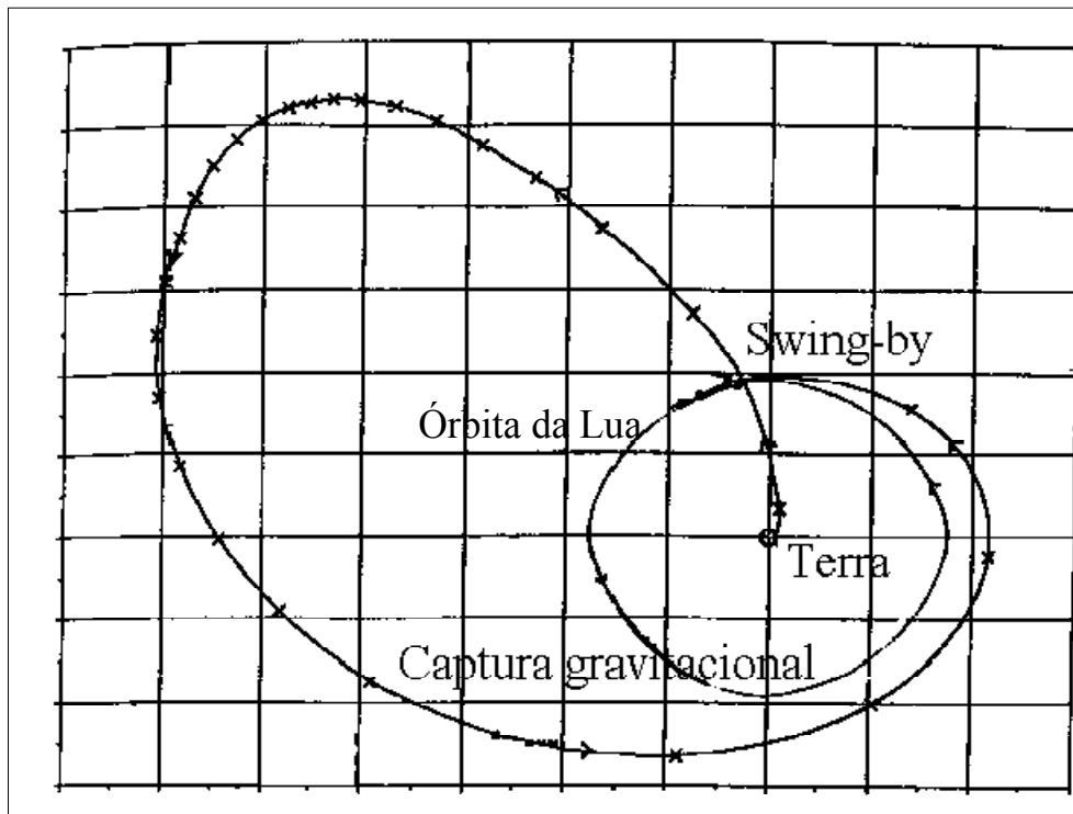
Fig. 9.1 – Transferência completa Terra-Lua.
