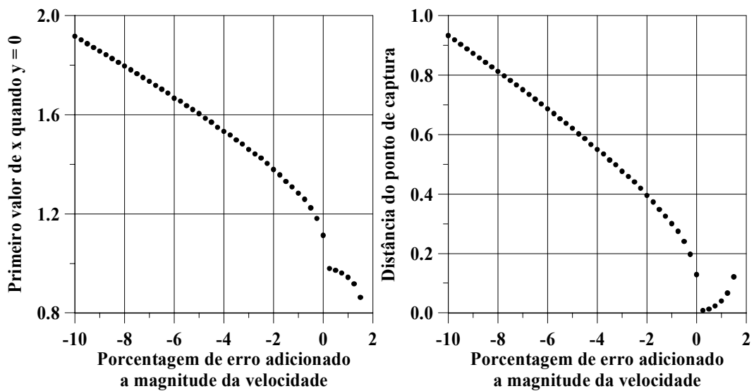
Fig. 9.5 – Resultados para erros de 10% na magnitude da velocidade.
