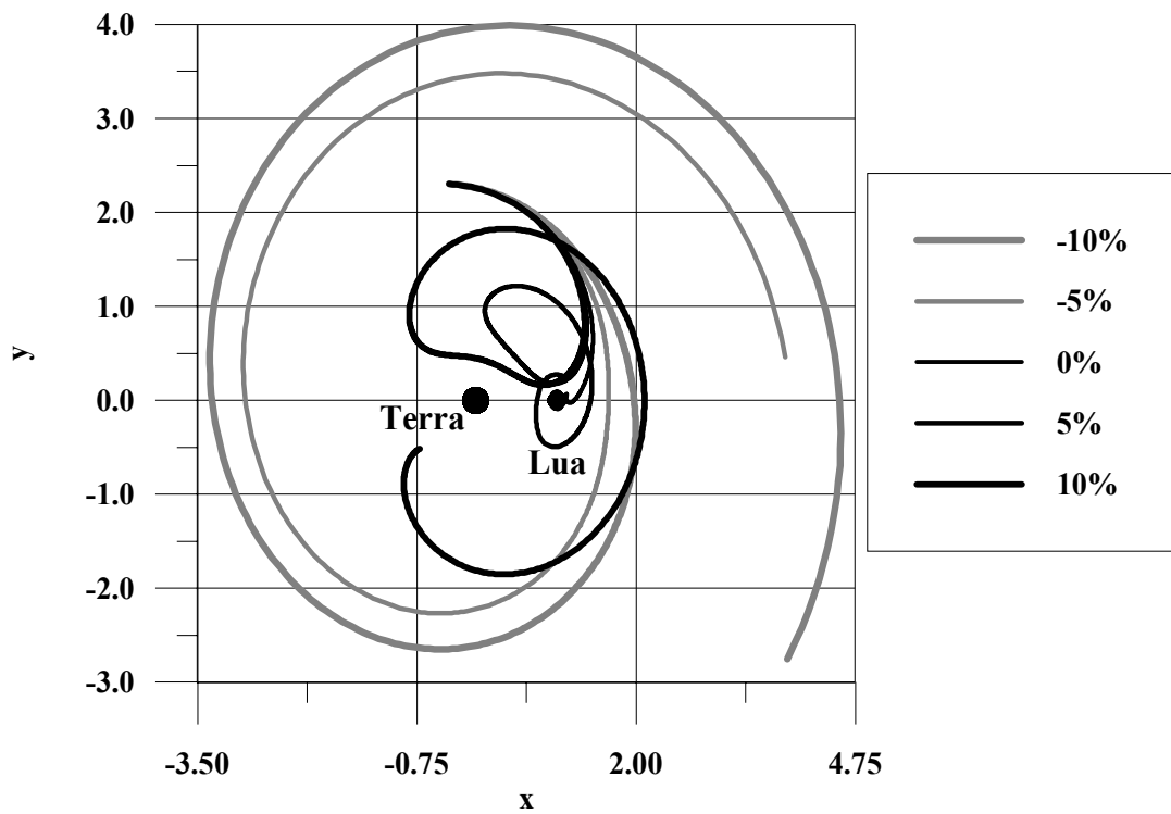
Fig. 9.14 – Trajetórias com erros na magnitude da velocidade.
