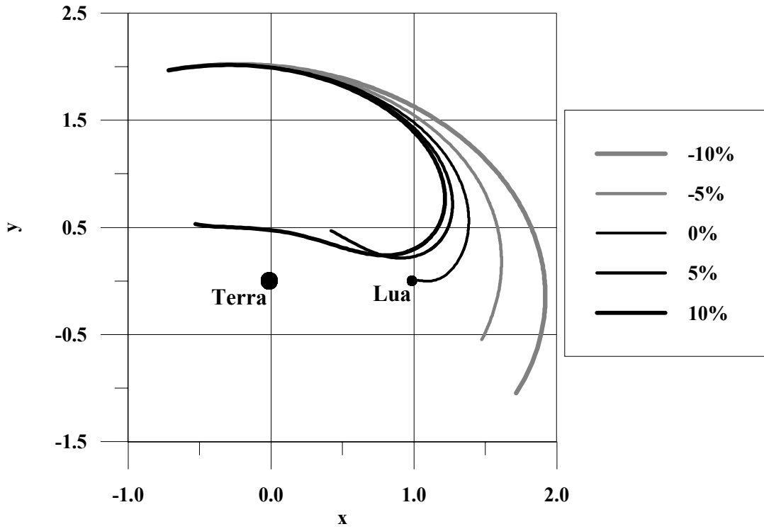
Fig. 9.4 – Trajetórias com erros na magnitude da velocidade.
