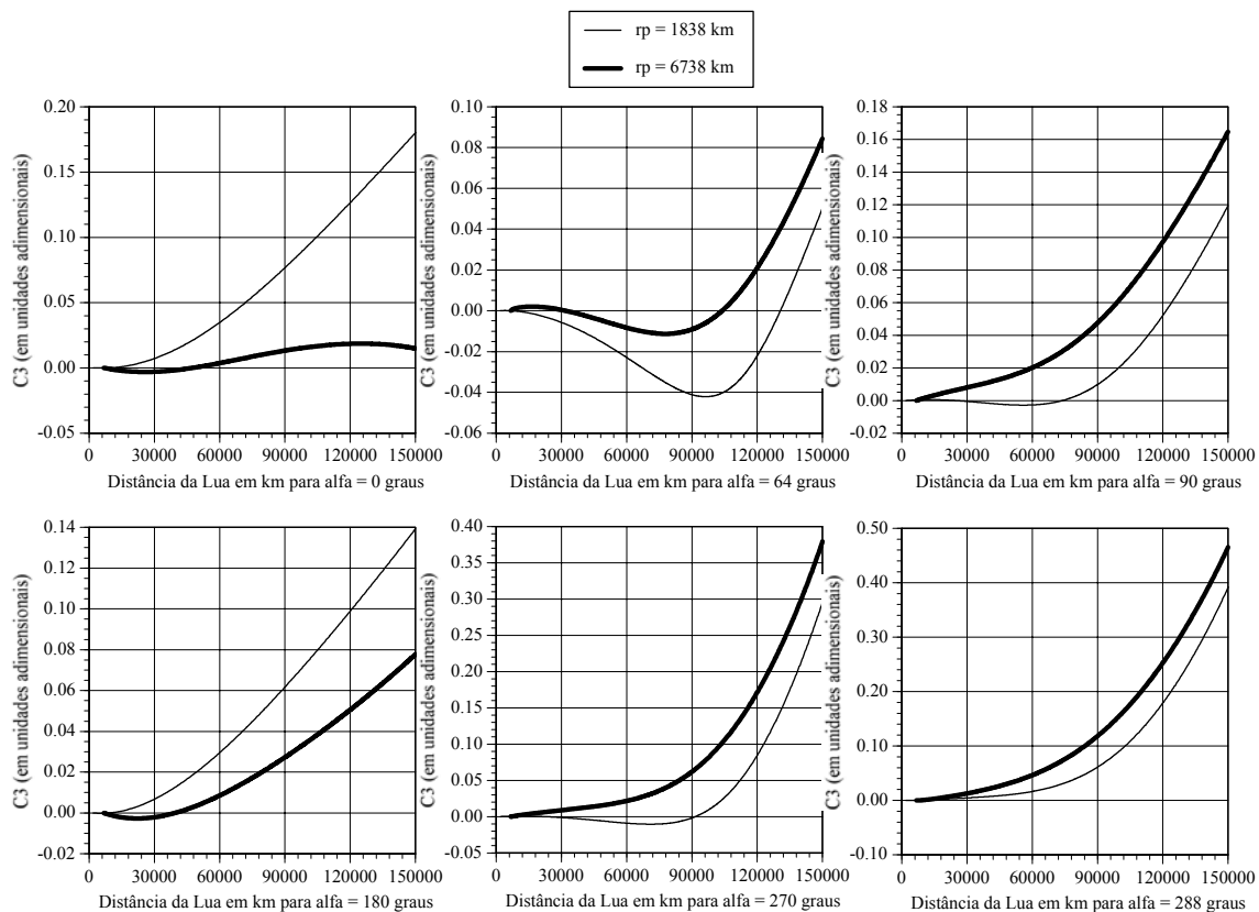
Fig. 4.1 – Comportamento de C_3 em relação à distância da Lua para o valor inicial C_3 = 0 .
