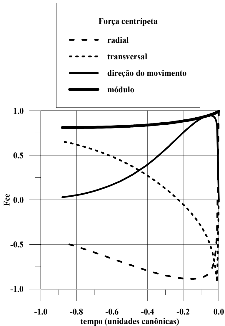
Fig. 5.35 – Força centrípeta para o terceiro caso.
