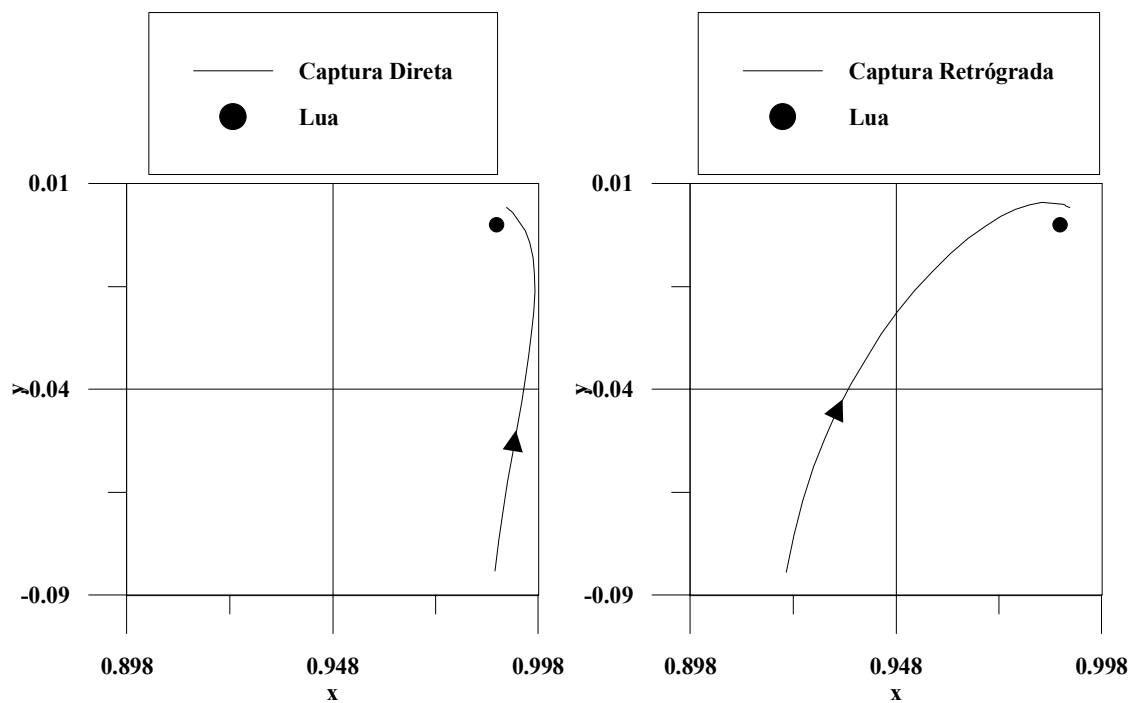
Fig. 2.5 – Magnificação das capturas da Figura 2.4.
