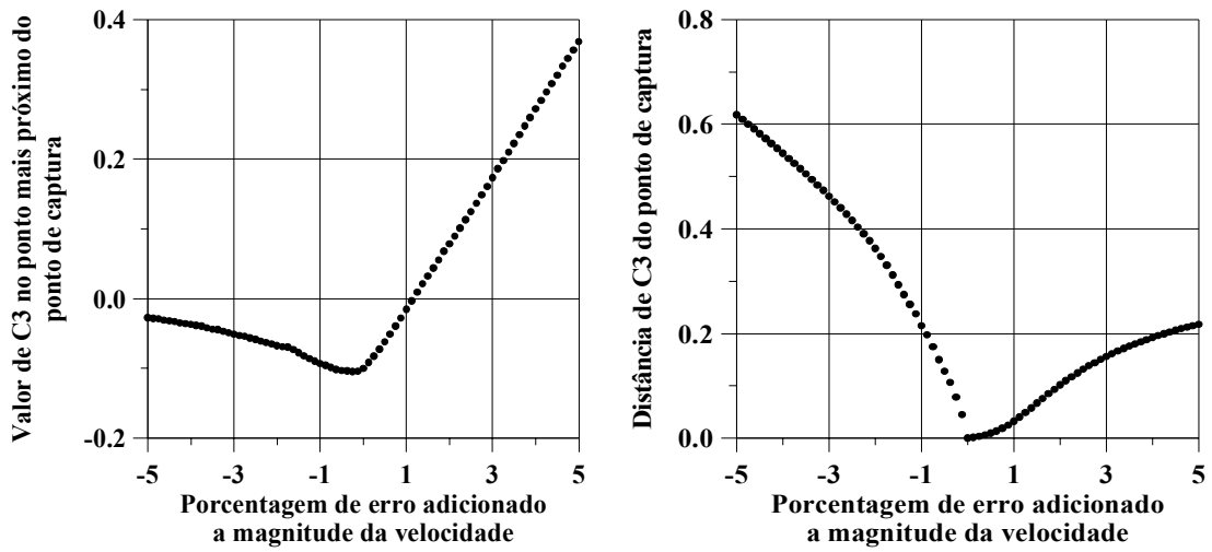
Fig. 9.8 – Resultados para erros de 5% na magnitude da velocidade.
