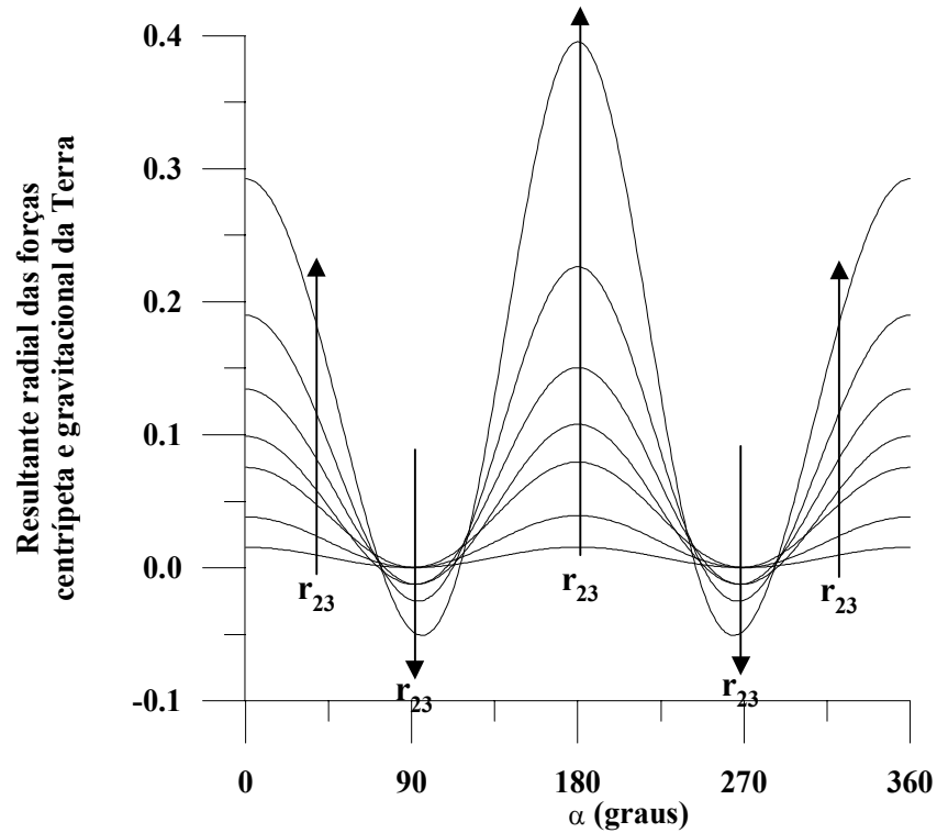
Fig. 5.11 –Força resultante das forças de gravidade devido a Terra e da centrípeta na direção radial.
