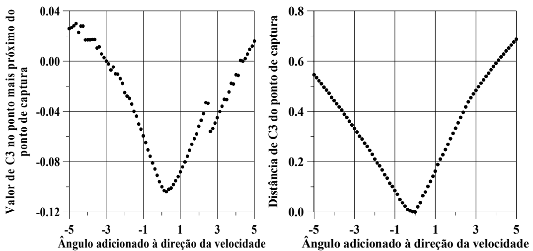
Fig. 9.21 – Resultados para erros de até 5^\circ na direção da velocidade.
