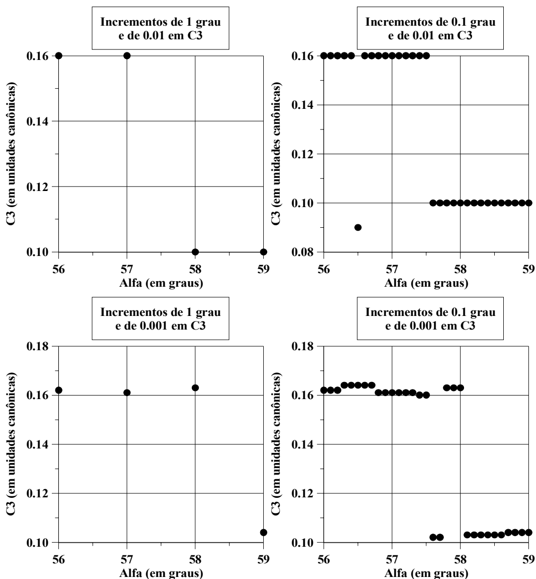
Fig. 6.2 – Ampliação da descontinuidade perto de 60°.
