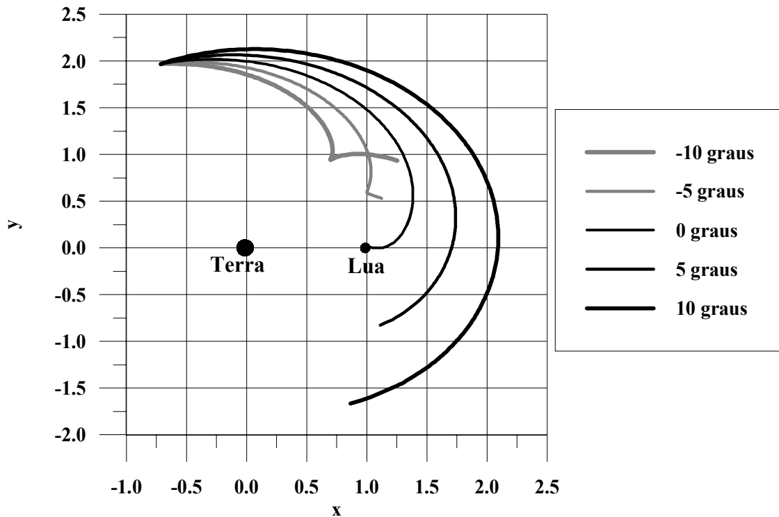
Fig. 9.17 – Trajetórias com erros na direção da velocidade.
