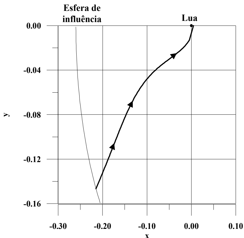
Fig. 5.14 – Trajetória com C3 = -0.15 e \alpha = 0^\circ .
