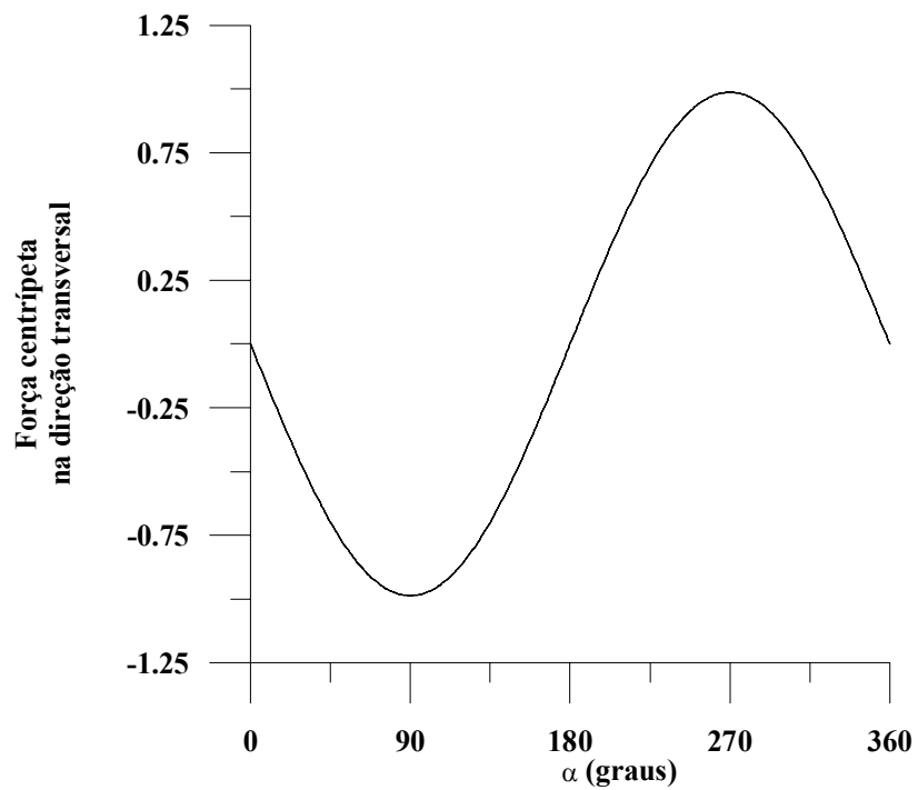
Fig. 5.8 – Força centrípeta na direção transversal.
