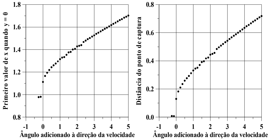
Fig. 9.20 – Resultados para erros de até 5^\circ na direção da velocidade.
