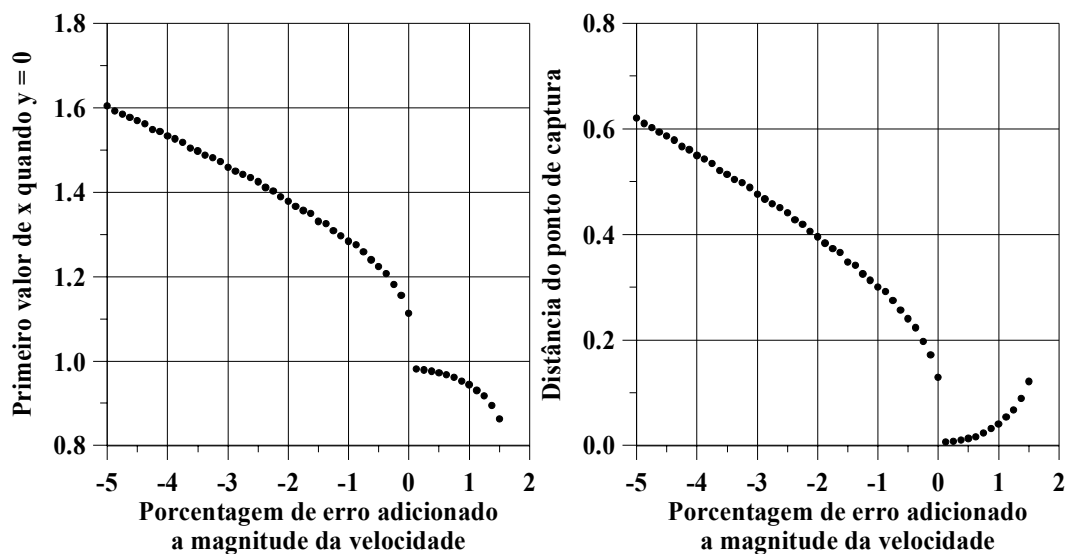
Fig. 9.7 – Resultados para erros de 5% na magnitude da velocidade.
