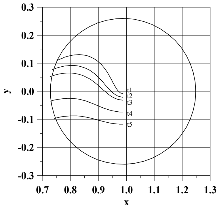
Fig. 7.8 – Trajetórias com C3 = -0.05 e \alpha = 270^\circ .
