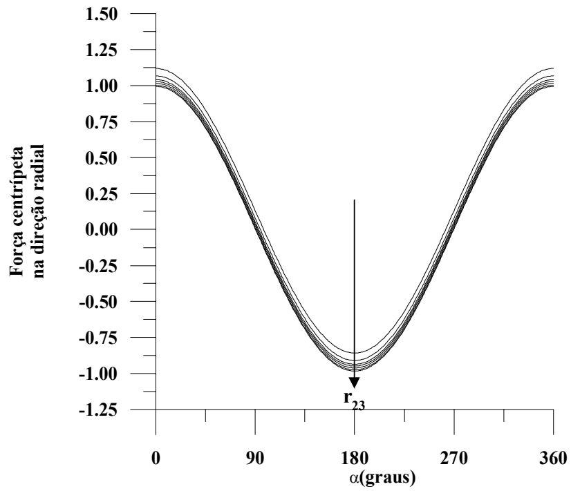
Fig. 5.7 – Força centrípeta na direção radial.
