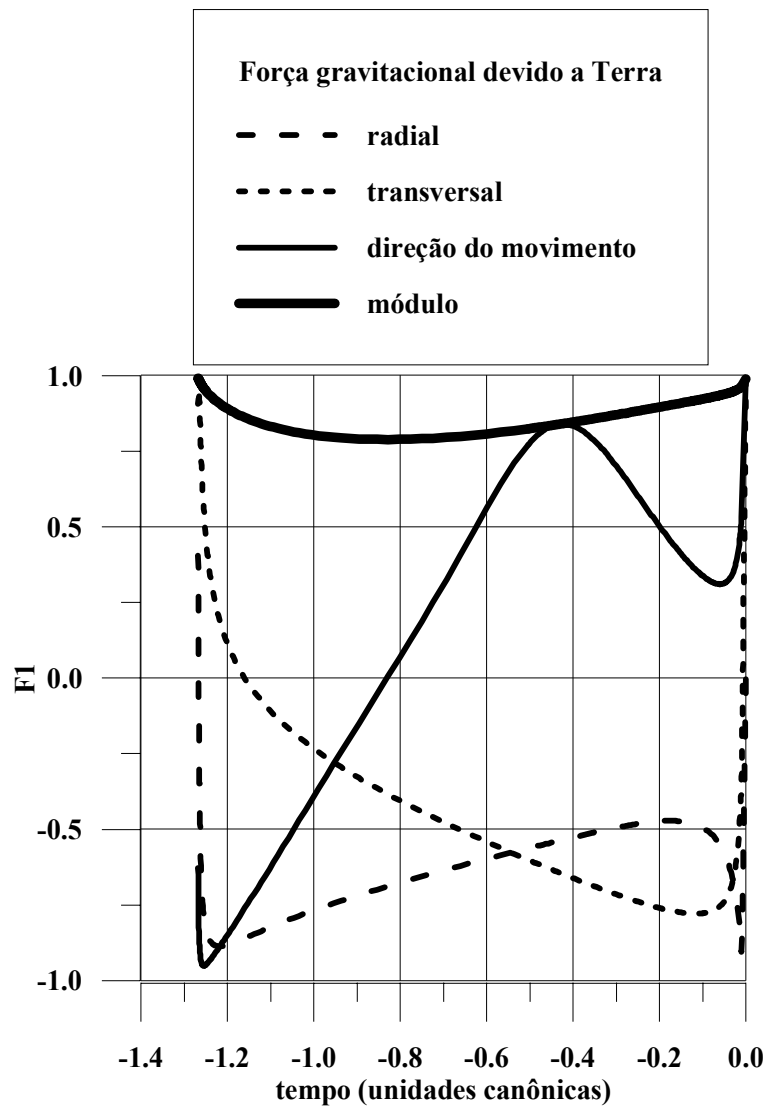
Fig. 5.27 – Força da gravidade da Terra para a terceira trajetória.
