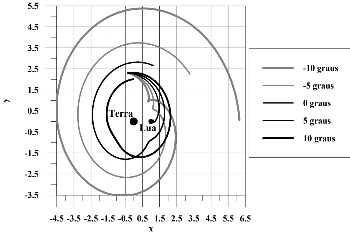
Fig. 9.27 – Trajetórias com erros na direção da velocidade.
