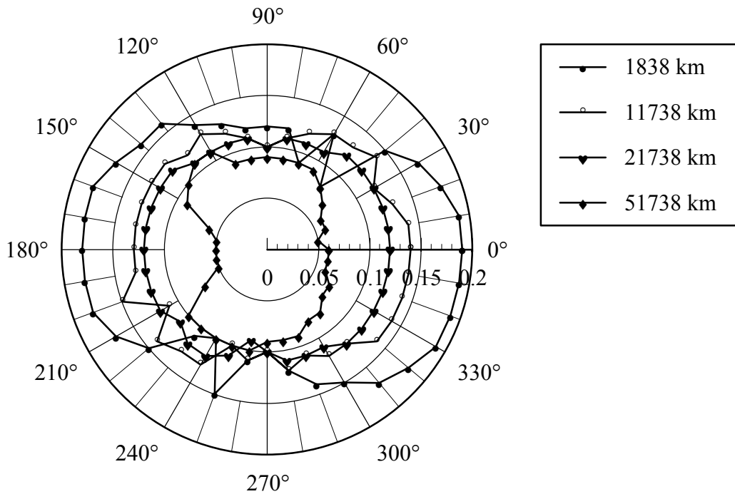
Fig. 6.5 – Valores mínimos de C_3 para vários r_p na captura retrógrada.
