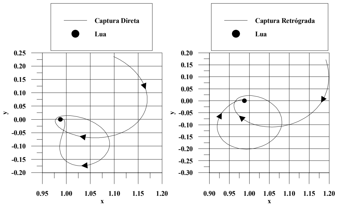
Fig. 2.4 – Capturas direta e retrógrada.
