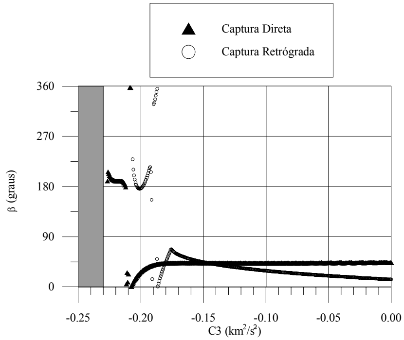
Fig. 3.5 – Ângulo da posição de entrada vs. C3 na periluna.
