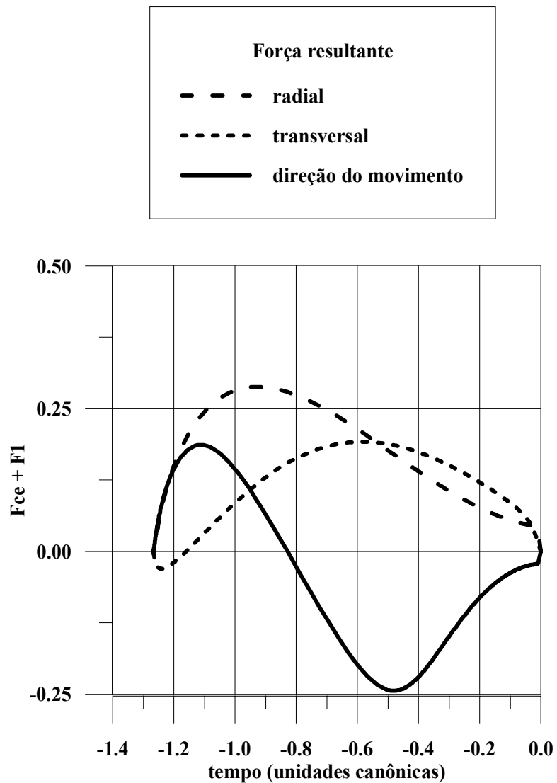
Fig. 5.30 – Força resultante para a terceira trajetória.
