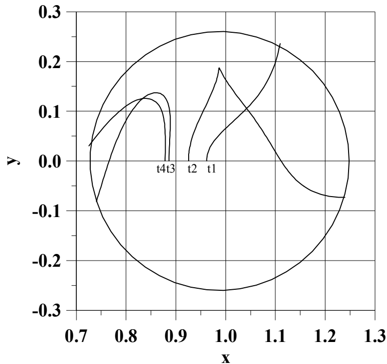
Fig. 7.7 – Trajetórias com C3 = -0.05 e \alpha = 180^\circ .
