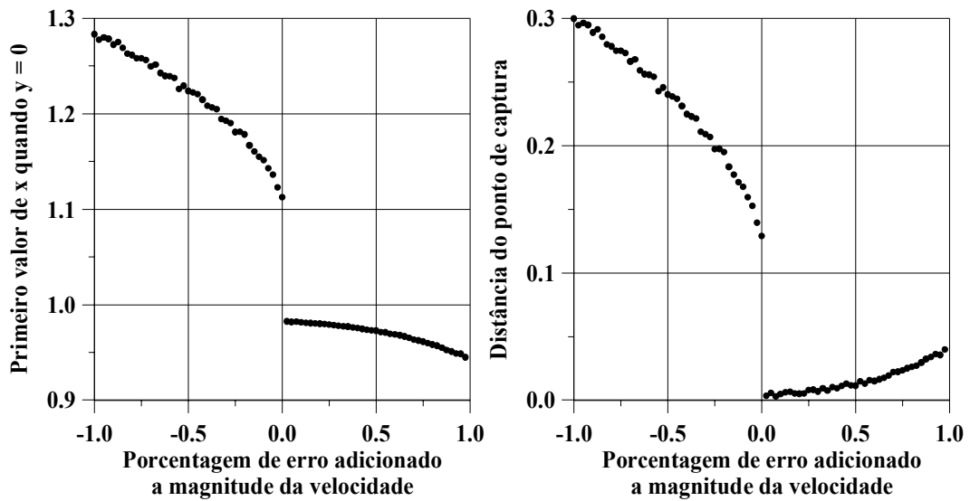
Fig. 9.9 – Resultados para erros de 1% na magnitude da velocidade.
