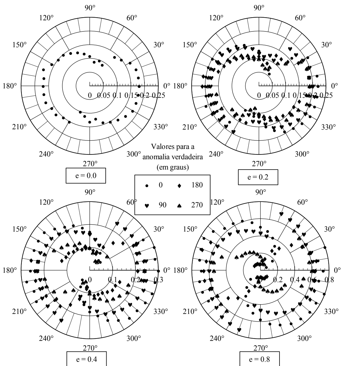
Fig. 8.6 – Comportamento da energia mínima para \mu = 0.01 e excentricidades variadas.
