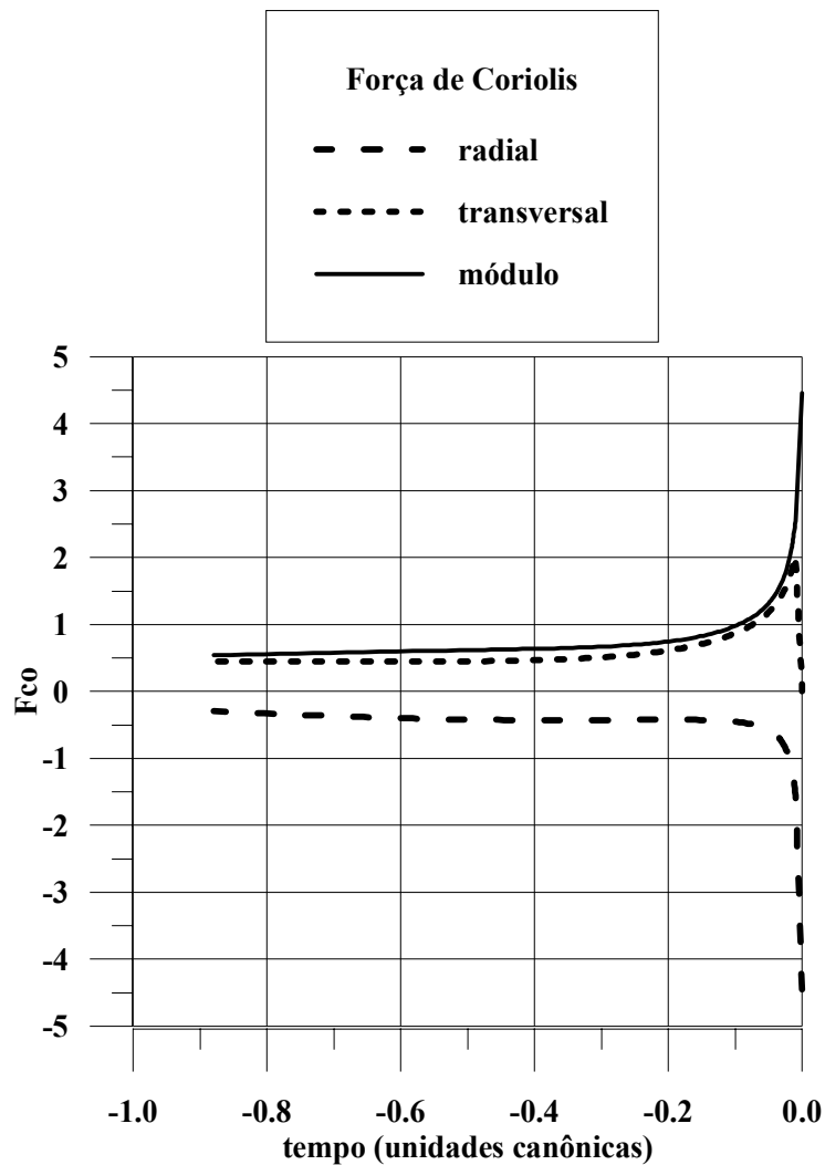
Fig. 5.37 – Comportamento da força de Coriolis na quarta trajetória.
