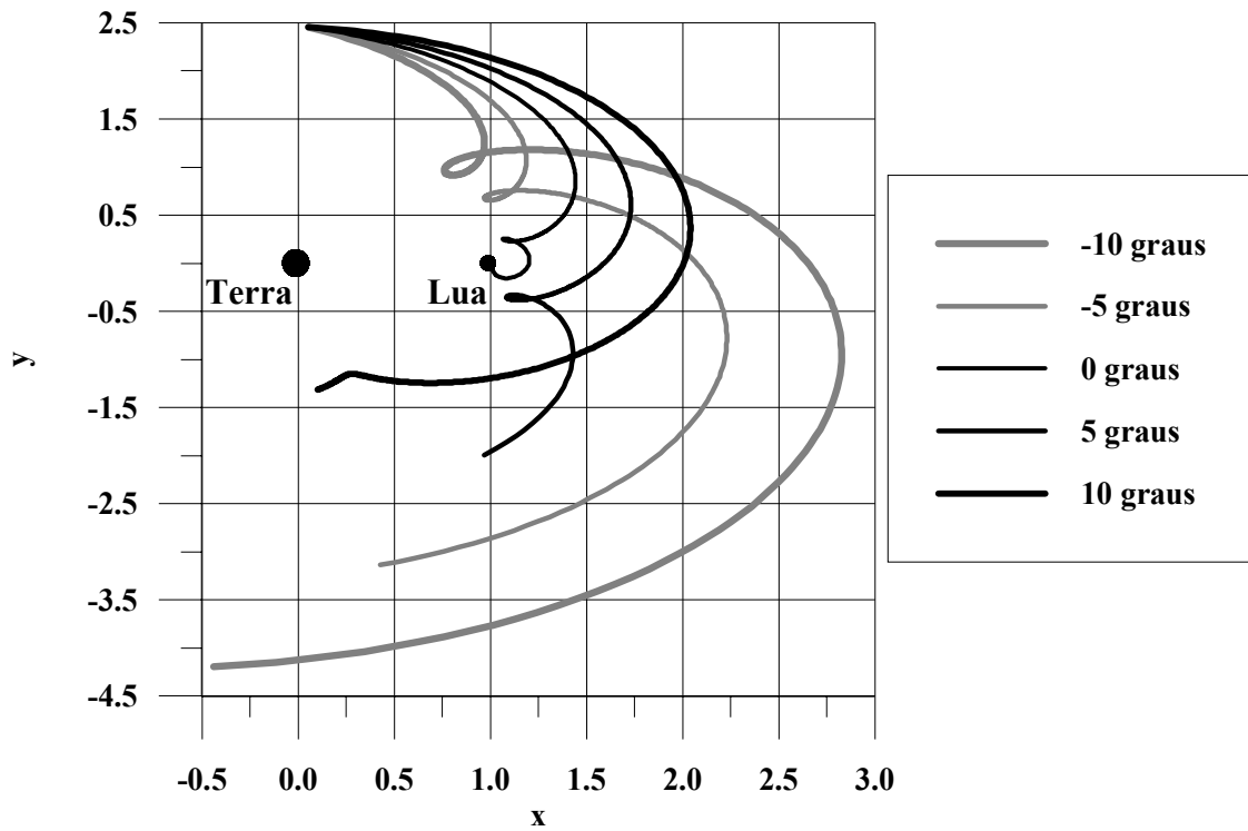
Fig. 9.24 – Trajetórias com erros na direção da velocidade.
