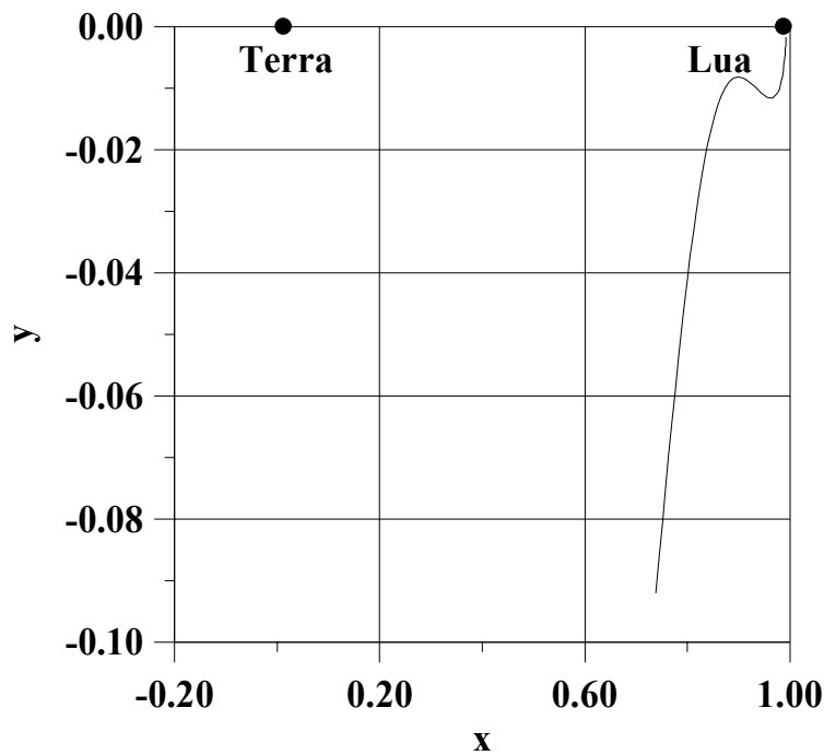
Fig. 8.9 – Trajetória do problema 1.
