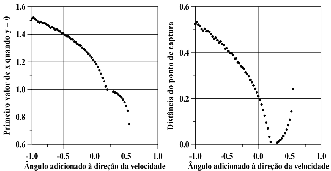
Fig. 9.25 – Resultados para erros de até 1^\circ na direção da velocidade.
