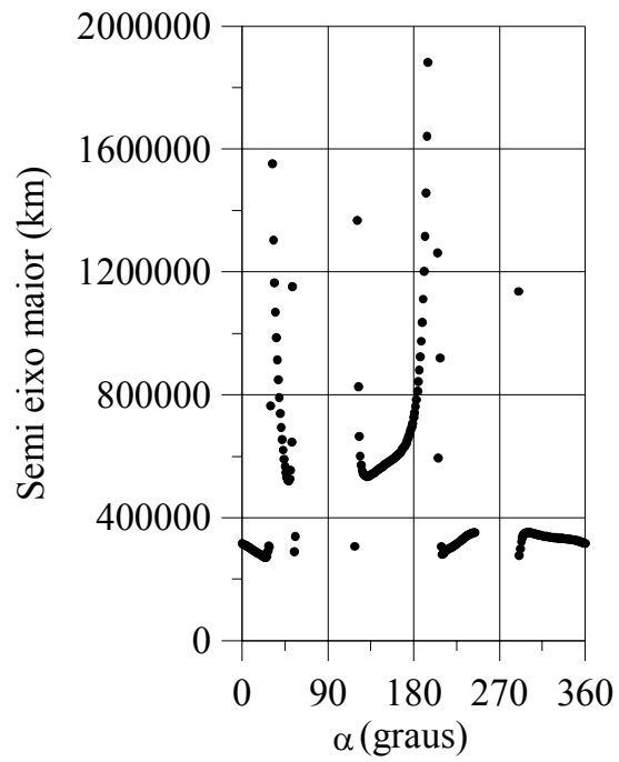
Fig. 3.11 – Semi-eixo maior vs. ângulo de posição da periluna.
