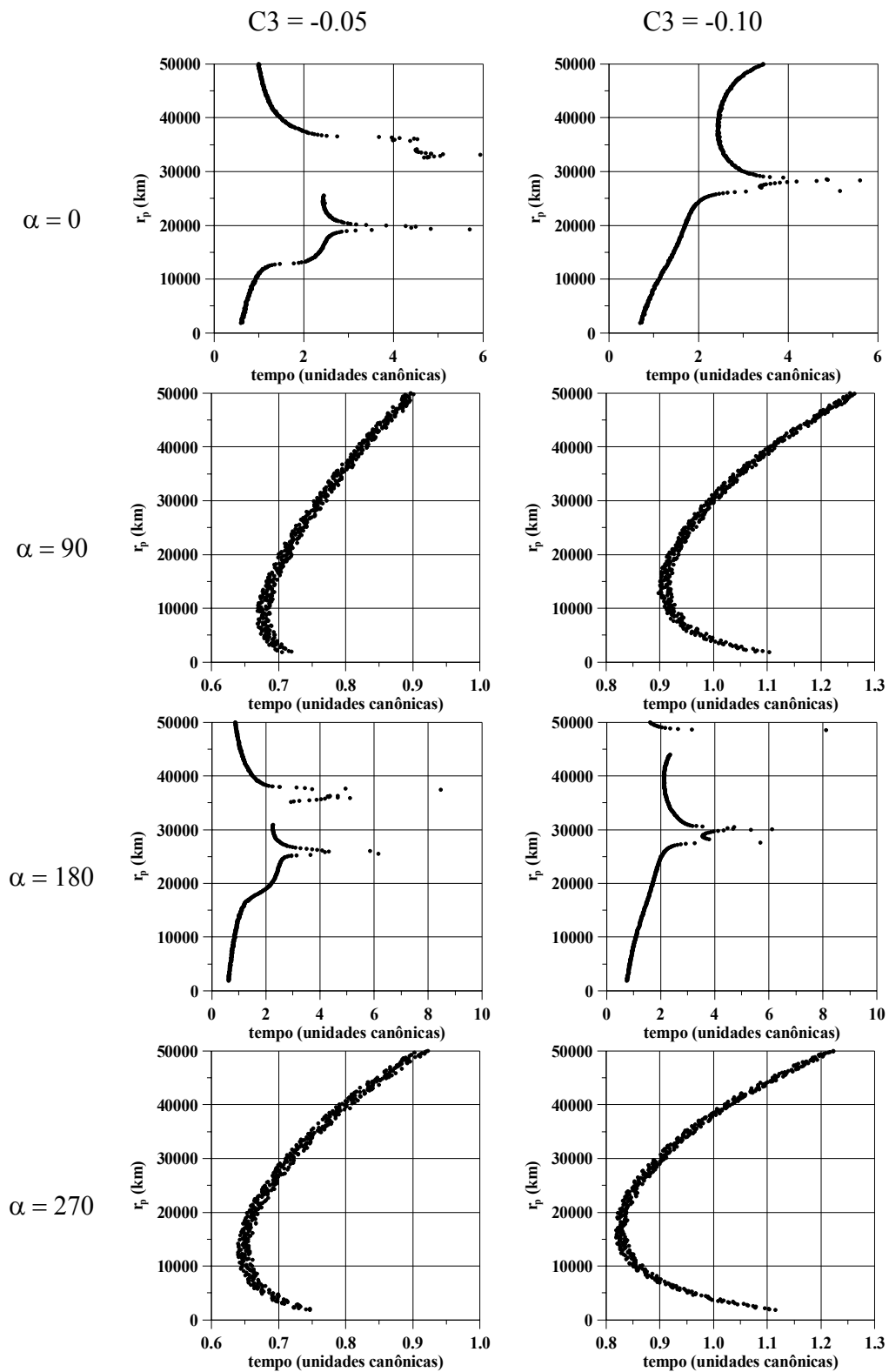
Fig. 7.6 – Periluna em função do tempo de captura.
