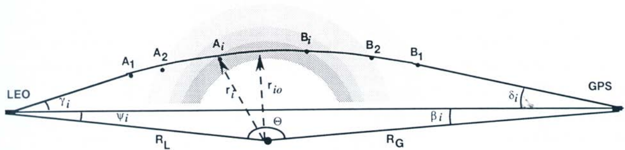
FIGURA 2.3 – O raio traçado através de uma atmosfera estratificada. O caminho do raio atravessa a i -ésima camada na sua melhor aproximação e os n_i são determinados seqüencialmente pela i -ésima observação Doppler e pelas condições de contorno, usando os valores de n previamente determinados para as camadas superpostas.
