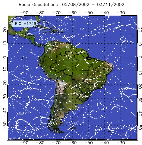
(a) Rádio Ocultações (RO)
