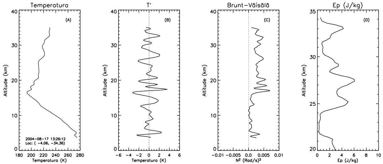
FIGURA 4.1 – (A) Perfil da temperatura observado no dia 17/08/2004 na região nordeste do Brasil ( 4,06^{\circ}S ; 34,36^{\circ}O ) em torno das 13:26 UT. (B) Flutuação da temperatura. (C) Freqüência de Brunt-Väisälä ao quadrado. (D) Energia potencial entre 20 e 35 km de altitude.
