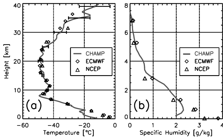
FIGURA 3.1 – Perfis verticais de (a) temperatura seca e (b) umidade específica calculadas a partir da ocultação número 5 em 11 de fevereiro de 2001 sobre o Atlântico Sul ( 53,2^{\circ}\text{S} ; 0,5^{\circ}\text{O} ; 19:43 UT) comparadas com dados do ECMWF e NCEP.
