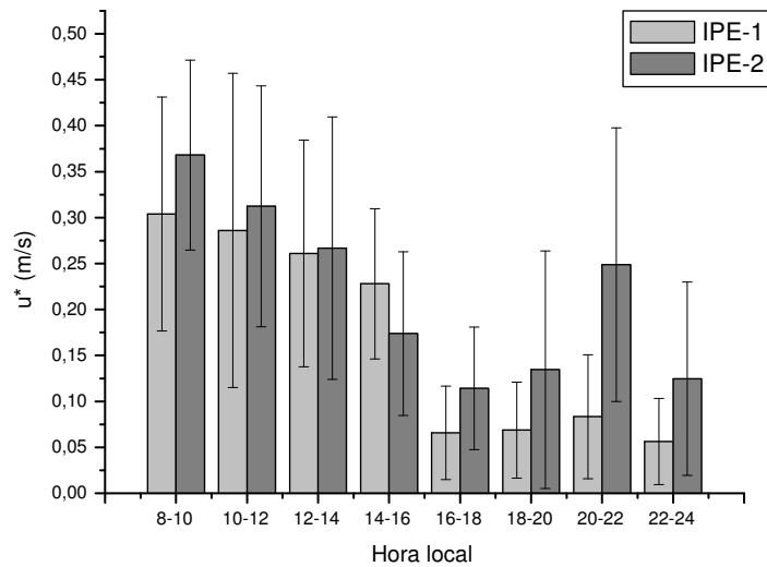
Fig. 5.20 – Variabilidade diurna de u_* para os experimentos IPE-1 e IPE-2
