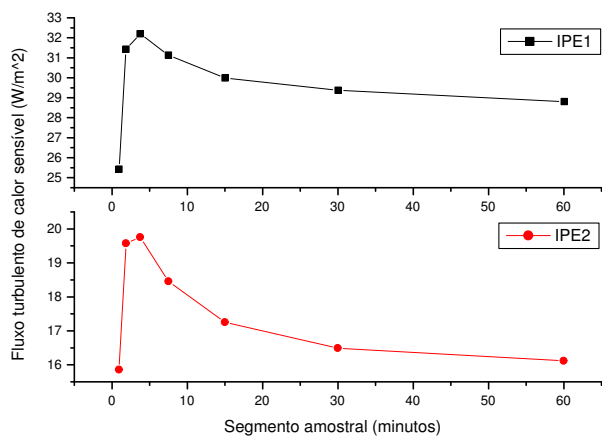
Fig. 4.11 – Comparação de H calculado para segmentos amostrais de diversos tamanhos, nos dois experimentos (média para todos os horários disponíveis): a) IPE-1; b) IPE-2
