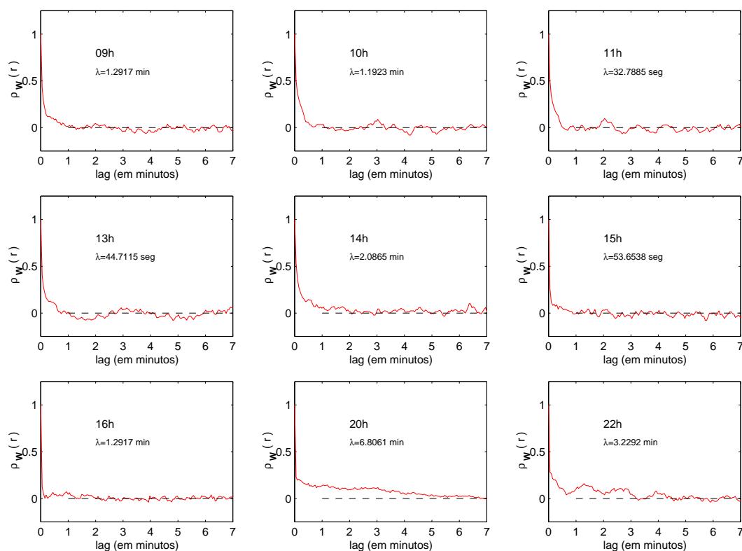
Fig. 5.4 – Função de autocorrelação para diversos horários do dia 143 do experimento IPE-1, para w , componente vertical da velocidade do vento.
