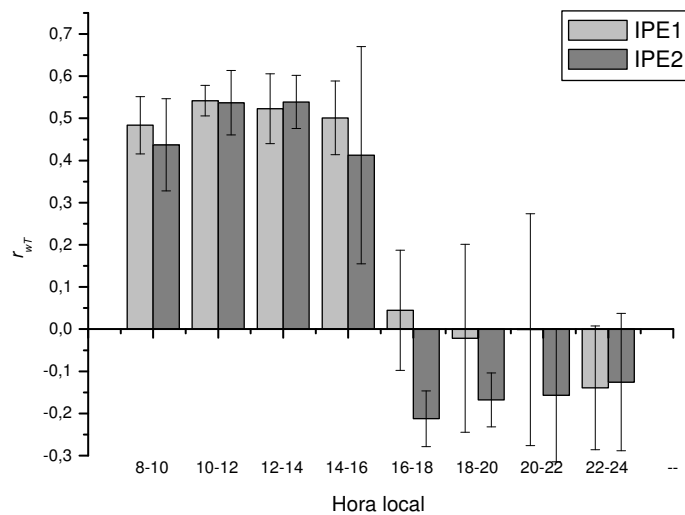
Fig. 5.10 – Evolução horária do coeficiente de correlação r_{wT} para os dois experimentos, IPE-1 e IPE-2.
