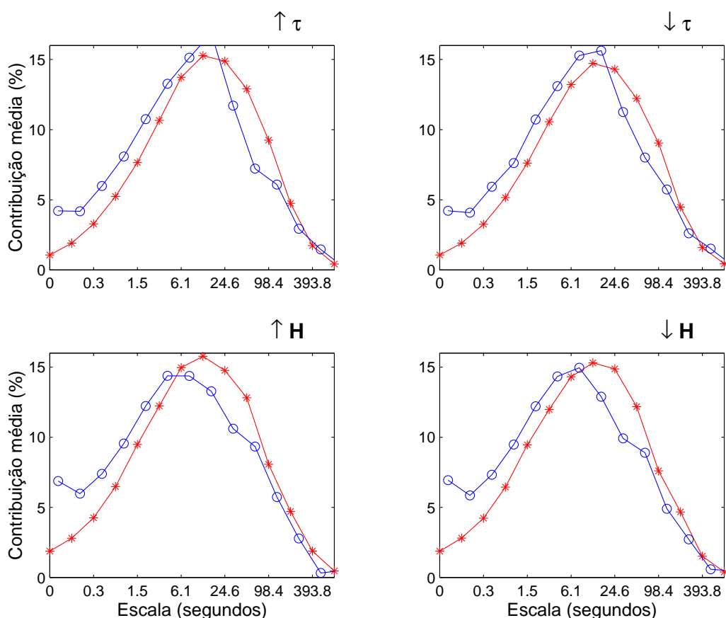
Fig. 5.31 – Contribuição de intrusões e ejeções para \tau e H na situação diurna. a) ejeção em \tau ; b) intrusão em \tau ; c) ejeção em H ; d) intrusão em H . Legenda: * – IPE-1; \circ – IPE-2
