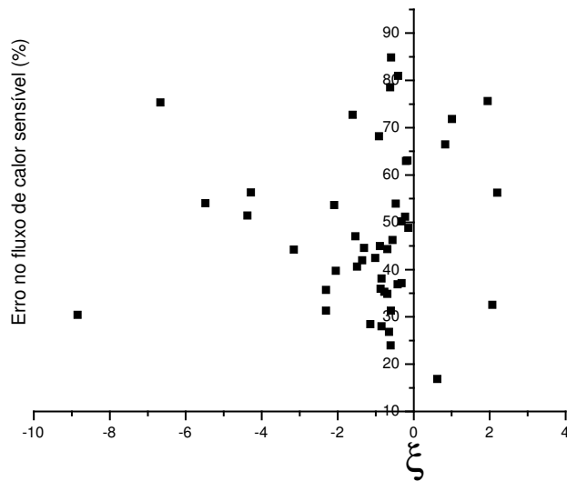
Fig. 5.16 – Variação do erro em H em função do parâmetro de estabilidade \xi para diversos horários do experimento IPE-1.
