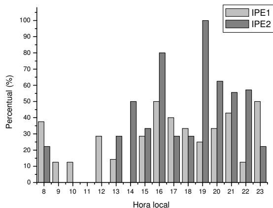
Fig. 4.4 – Distribuição dos horários em que predominam condições não-estacionárias, para cada uma das duas campanhas no Pantanal
