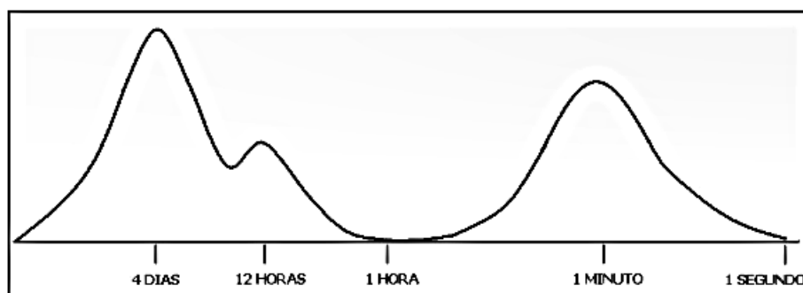
Fig. 4.5 – Idealização do espectro da velocidade do vento para uma larga banda de escalas temporais (variância da velocidade do vento no eixo vertical e escala temporal no eixo horizontal). FONTE: Adaptada de Stull (1988).
