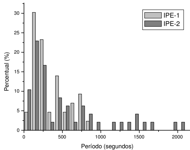
Fig. 5.7 – Distribuição dos valores de \lambda_u para a faixa de horários de 8 às 15 horas nos experimentos IPE-1 e IPE-2
