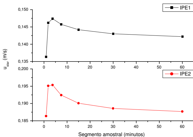
Fig. 4.12 – Comparação do valor de u_* calculado para segmentos amostrais de diversos tamanhos, nos dois experimentos (média para todos os horários disponíveis): a) IPE-1; b) IPE-2
