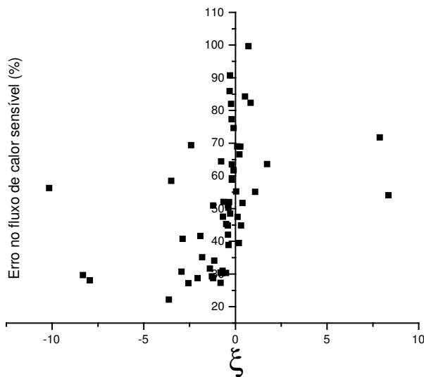
Fig. 5.17 – Variação do erro em H em função do parâmetro de estabilidade \xi para diversos horários do experimento IPE-2.
