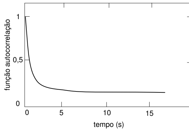
Fig. 5.3 – Função autocorrelação de um sinal com escalas muito maiores do que as turbulentas, tendências lineares, por exemplo. FONTE: Adaptação de Lumley e Panofsky (1964).
