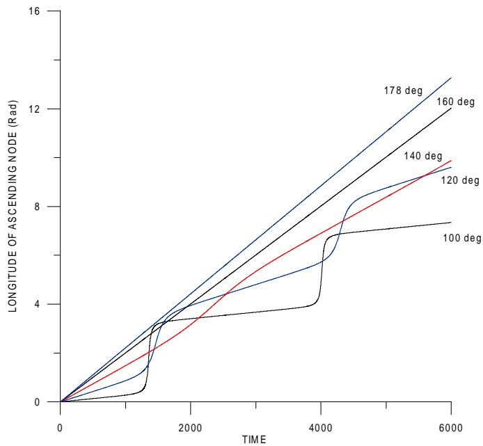
Figure. 7- Evolution of the longitude of ascending node.
