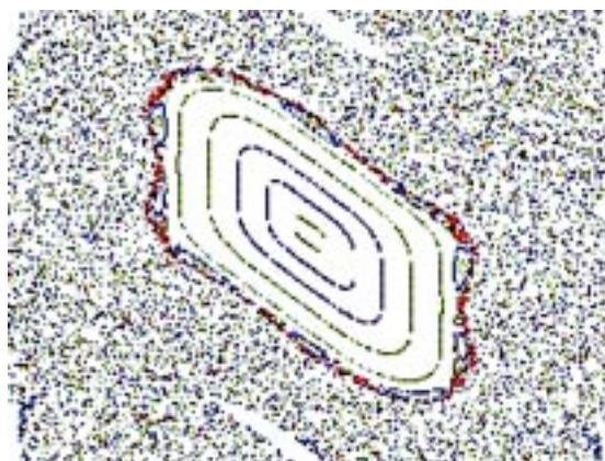
Figura 6. Espaço de fase representando um sistema com características similares às que estão presentes nos problemas envolvendo a reorientação de naves espaciais. Cada trajetória associada a uma diferente condição inicial – no caso da nave, posição e velocidade – aparece representada por pontos de cores diferentes. A região de alta densidade está associada a uma única trajetória caótica que preenche densamente o espaço que a envolve, expressão da propriedade transitiva. Note-se que existem outras trajetórias que não apresentam uma dinâmica caótica (região central da figura)
