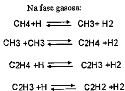
Figura 5 – Algumas reações que ocorrem na região do raio crítico na fase gasosa
