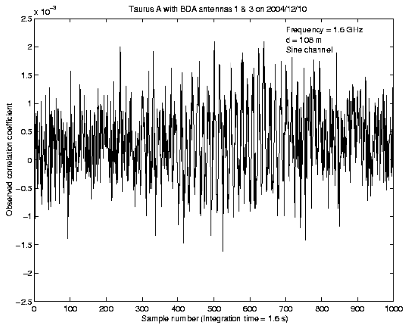
FIGURA A.12 - Franja seno obtida em 10/12/2004 pelo par interferométrico composto pelas antenas A1 e A3 na observação de Taurus A.
