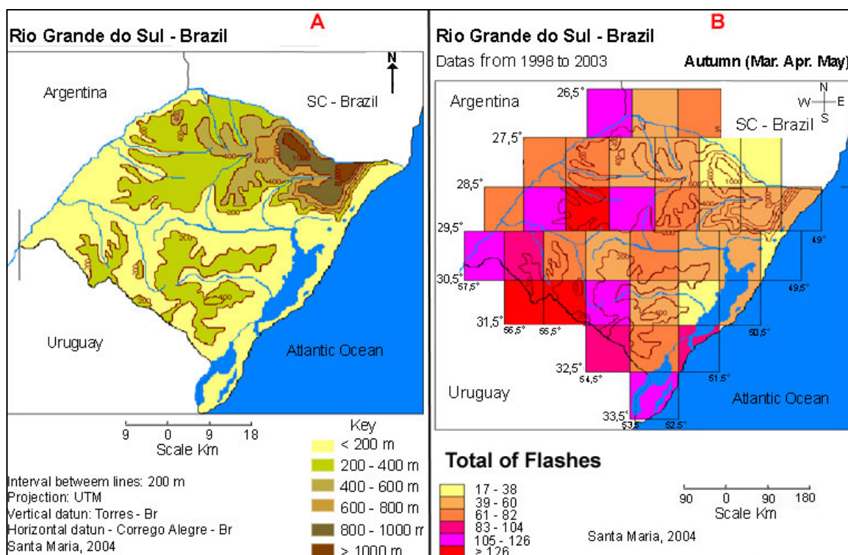
Figura 51 – A) Relevo do Rio Grande do Sul. B) Distribuição média de relâmpagos no Rio Grande do Sul, 1998 a 2003, com base em dados do sensor LIS.
