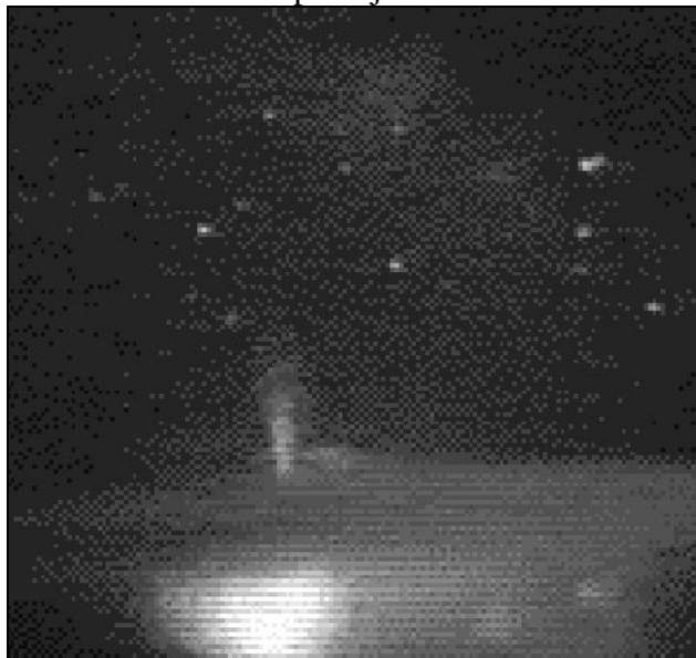
FIGURA 52 – Jatos azuis, blue jats em preto e branco Fonte: Sentman (1998) e Tavares (1999, p. 49 e 50)
