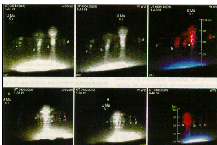
Figura 32 – Imagem dos sprites .
