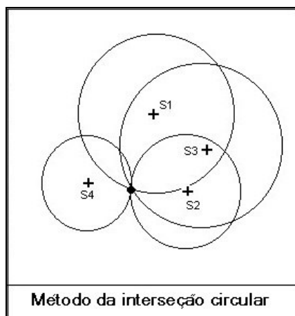
Figura 37 – Método das interseções circulares.
