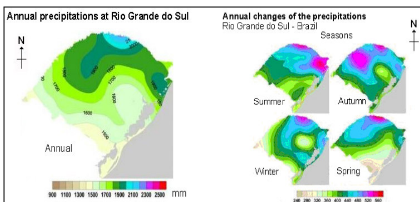
Figura 54 – Média das precipitações sazonais e anuais.
