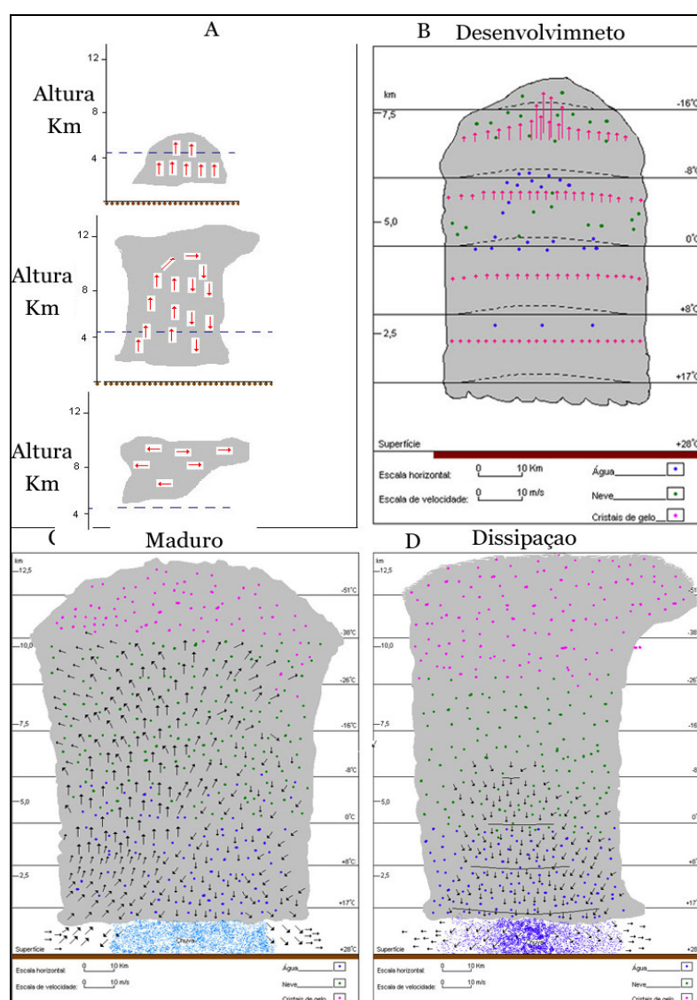
Figura 5 – A – Estágios de uma tempestade unicelular
