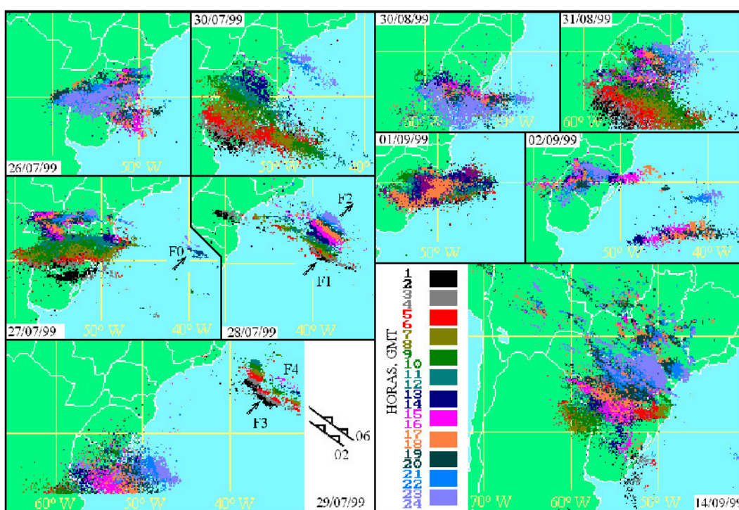
Figura 57 – Campos Acumulados das Descargas durante ciclogênese local.
