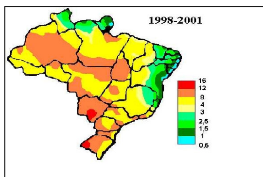
Figura 50 – Mapa de densidade de relâmpagos do Brasil.
