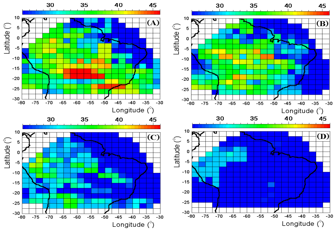
Figura 14 – Imageamento dos albedo máximos estimados pelo ECS2 para os períodos do sexto bimestre de 1998 (A), do primeiro (B), do segundo (C) e do terceiro bimestre de 1999 (D).
