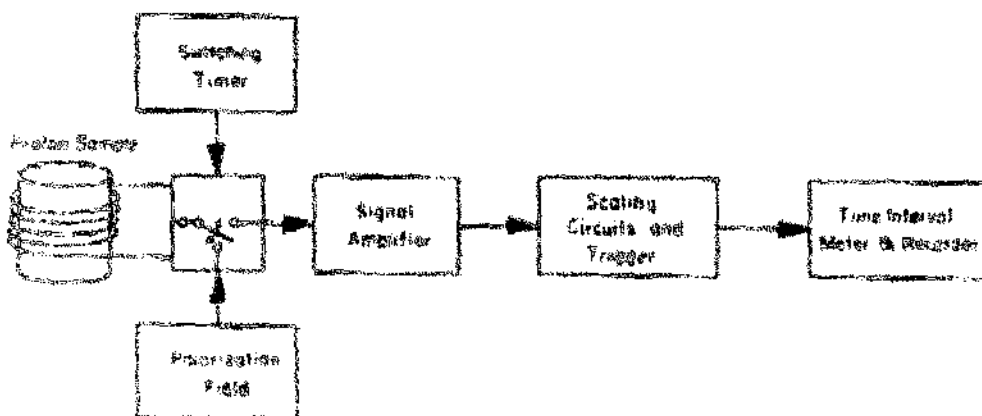
Figura 4-2 – Magnetômetro de próton para medida do Campo Geomagnético total. A bobina ao redor da amostra é utilizada para alinhar os prótons e detectar o período de precessão dos mesmos. (Campbell, 1997)
