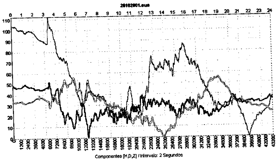
Anexo 10 (a-b) - Variação nas componentes H - Verde -, D - Azul - e Z - Vermelho - do Campo Magnético Terrestre, para as Estações Magnéticas de São Martinho da Serra - SMS - e Eusébio - EUS -, SMS vista em três dimensão e EUS vista em uma dimensão, referente ao dia 28102001.
