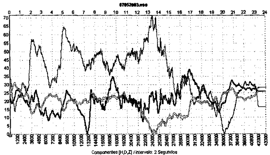
Anexo 6 (a-b) - Variação nas componentes H - Verde -, D - Azul - e Z - Vermelho - do Campo Magnético Terrestre, para as Estações Magnéticas de São Martinho da Serra - SMS - e Vassouras - VSS -, dia de uma Tempestade Magnética, referente ao dia 07052003.
