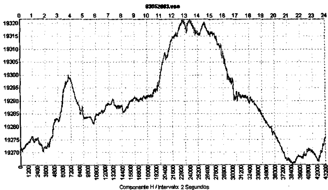
Anexo 4 (a-b) - Variação na componente H do Campo Magnético Terrestre, para as Estações Magnéticas de São Martinho da Serra - SMS - e Vassouras - VSS -, referente ao dia 03052003.
