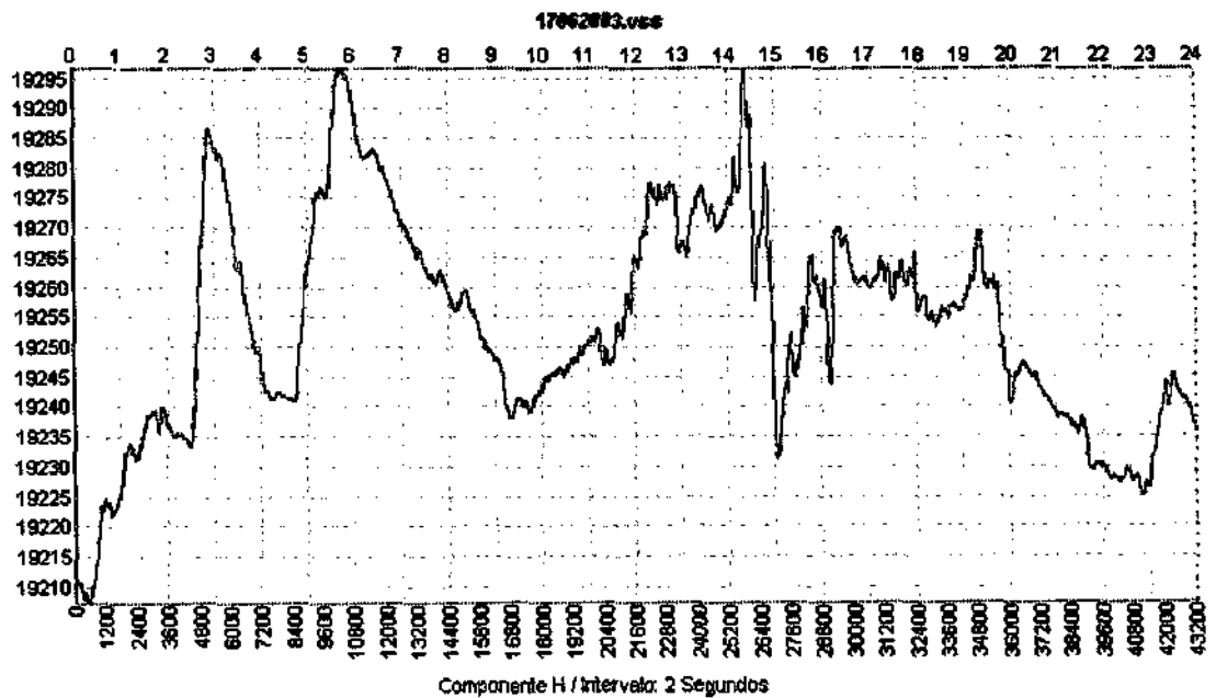
Anexo 8 (a-b) - Variação na componente H do Campo Magnético Terrestre, para as Estações Magnéticas de São Martinho da Serra - SMS - e Vassouras - VSS -, pulsação Impulsiva antecedendo uma Tempestade Magnética, referente ao dia 17062003.
