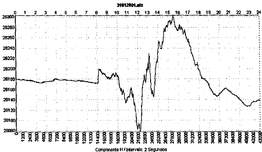
Anexo 13 (a-b) - Variação na componente H do Campo Magnético Terrestre, para as Estações Magnéticas de São Martinho da Serra - SMS - e São Luiz - SLZ -, pulsação Impulsiva, referente ao dia 31012001.
