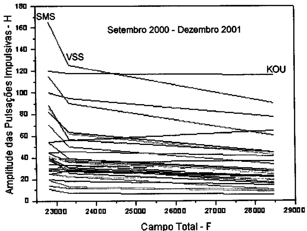
Figura 5-1- Estatística de pulsções Impulsivas para as Estações Magnéticas de São Martinho da Serra - SMS -, Vassouras - VSS -, Korou - KOU.
