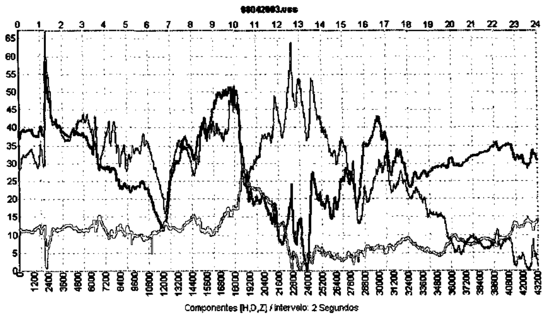
Anexo 3 (a-b) - Variação nas componentes H - Verde -, D - Azul - e Z - Vermelho - do Campo Magnético Terrestre, para as Estações Magnéticas de São Martinho da Serra - SMS - e Vassouras - VSS -, referente ao dia 08042003.
