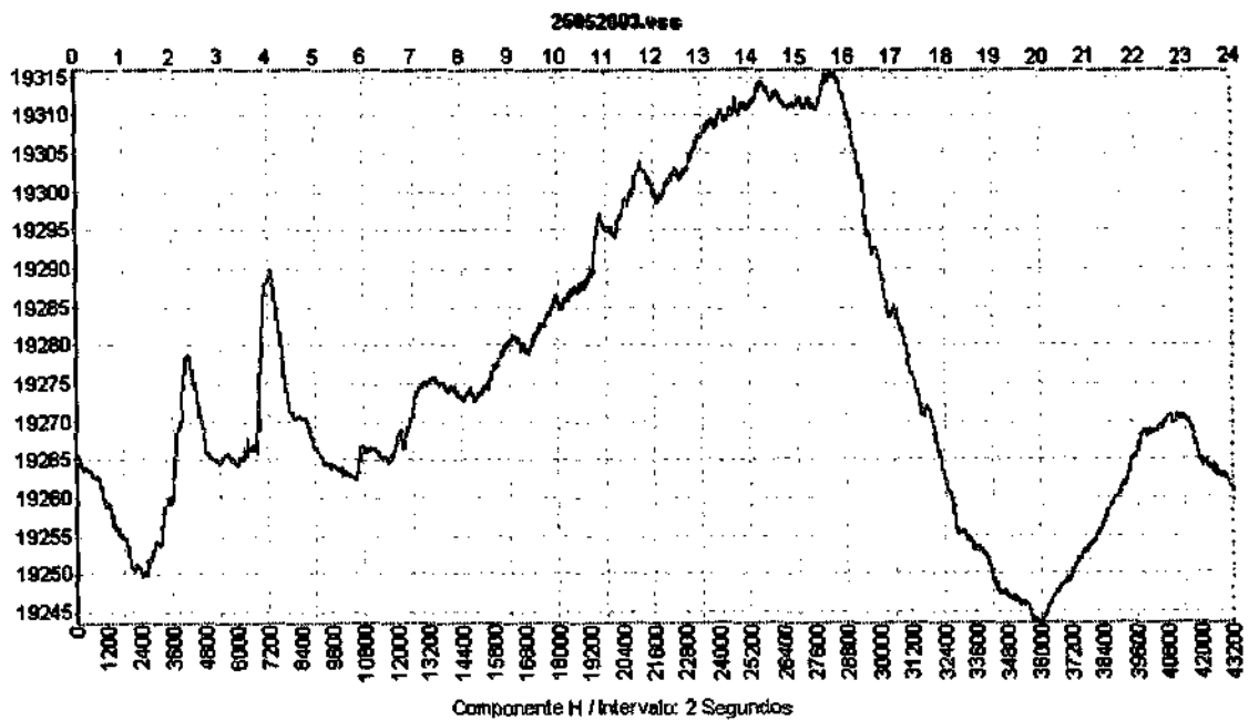
Anexo 5 (a-b) - Variação na componente H do Campo Magnético Terrestre, para as Estações Magnéticas de São Martinho da Serra - SMS - e Vassouras - VSS -, referente ao dia 25052003.
