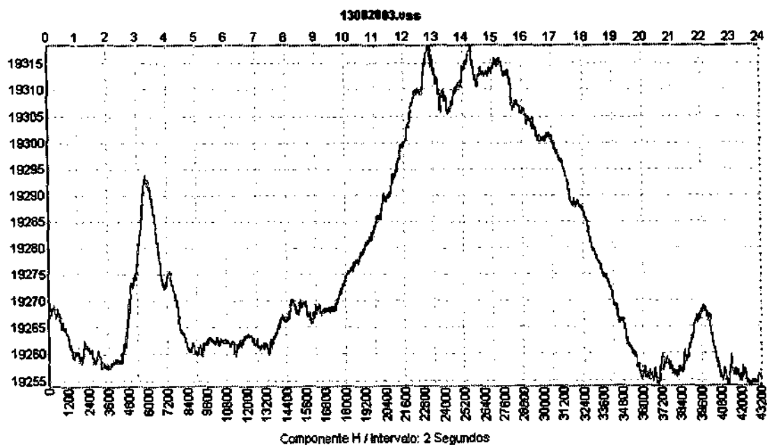
Anexo 11 (a-b) - Variação na componente H do Campo Magnético Terrestre, para as Estações Magnéticas de São Martinho da Serra - SMS - e Vassouras - VSS -, pulsação impulsiva, referente ao dia 13082003.
