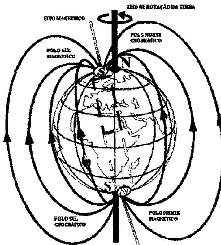
Figura 3 -1 - Dipolo Magnético colocado no centro da Terra e levemente inclinado em relação ao eixo de rotação. (Pinto e Gonzales, 1989)
