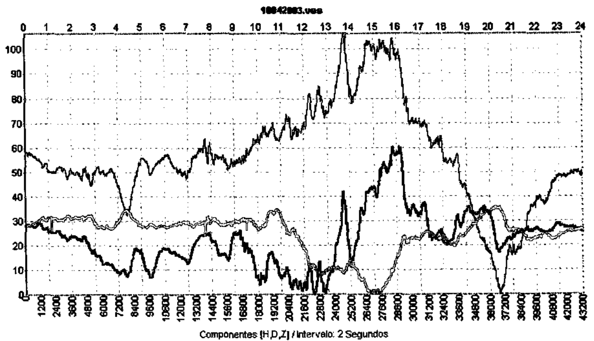
Anexo 1 (a-b) - Variação nas componentes H - Verde -, D - Azul - e Z - Vermelho - do Campo Magnético Terrestre, para as Estações Magnéticas de São Martinho da Serra - SMS - e Vassouras - VSS -, referente ao dia 10042003.
