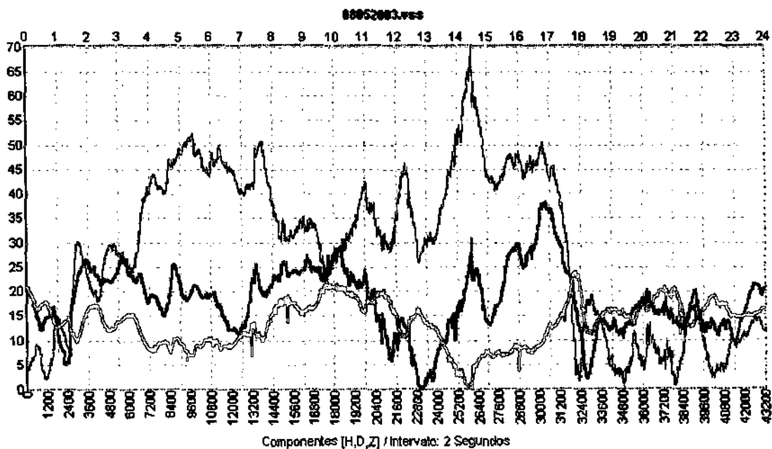
Anexo 7 (a-b) - Variação nas componentes H - Verde -, D - Azul - e Z - Vermelho - do Campo Magnético Terrestre, para as Estações Magnéticas de São Martinho da Serra - SMS - e Vassouras - VSS -, continuação da Tempestade Magnética, referente ao dia 08052003.
