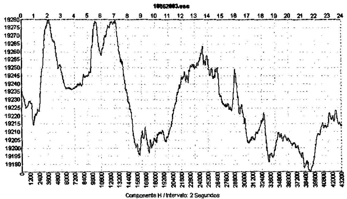
Anexo 9 (a-b) - Variação na componente H do Campo Magnético Terrestre, para as Estações Magnéticas de São Martinho da Serra - SMS - e Vassouras - VSS -, pulsação Impulsiva, referente ao dia 18062003.
