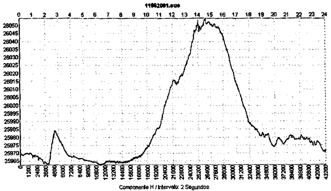
Anexo 12 (a-b) - Variação na componente H do Campo Magnético Terrestre, para as Estações Magnéticas de São Martinho da Serra - SMS - e Eusébio - EUS -, pulsação Impulsiva, referente ao dia 11062001.
