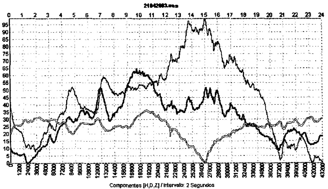
Anexo 2 (a-b) - Variação nas componentes H - Verde -, D - Azul - e Z - Vermelho - do Campo Magnético Terrestre, para as Estações Magnéticas de São Martinho da Serra - SMS - e Vassouras - VSS -, referente ao dia 21042003.
