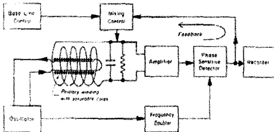
Figura 4-1 – Magnetômetro Fluxgate para medida direcional do Campo Geomagnético. (Campbell, 1997)
